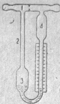
Рис. 8. Реометр с диафрагмой (Аркадьева).
