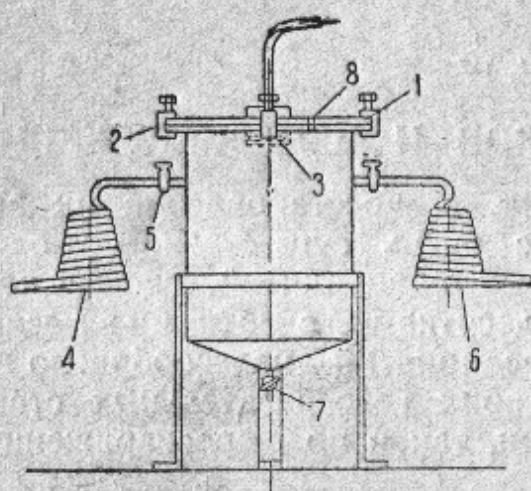
Рис. 23. Прибор для регенерации противогозовой коробки.
