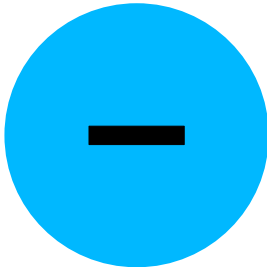
Elektrisch stark negativ geladener Körper
