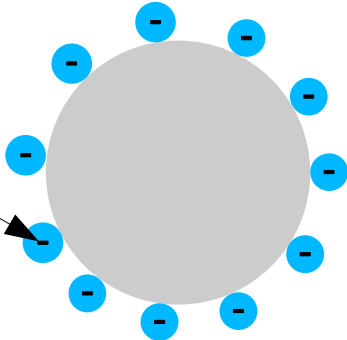
Körper mit beweglichen Oberflächenladungen
