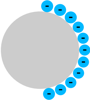
Oberflächenladungen werden verschoben
