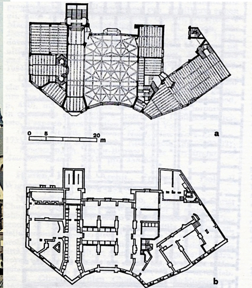
V. Horta. Bruxelles, maison du Peuple, 1895-99; a pianta del piano terra; b pianta del primo piano.
