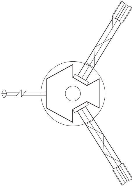
Abbildung 15: Aufsicht der "Yo-Yo"-Sonde (Skizze) [17]
