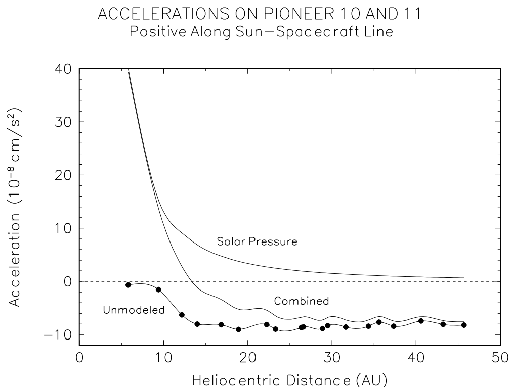
Abbildung 14: Die obere Kurze zeigt den Verlauf des Strahlungsdrucks, die untere die der Anomalie, in der Mitte die Kombination von beiden. Die Grafik erschien erstmals in [16]
