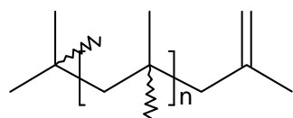
Hofmann-Produkt (~80 %)
