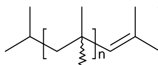
Zaitsev-Produkt (~20 %)
