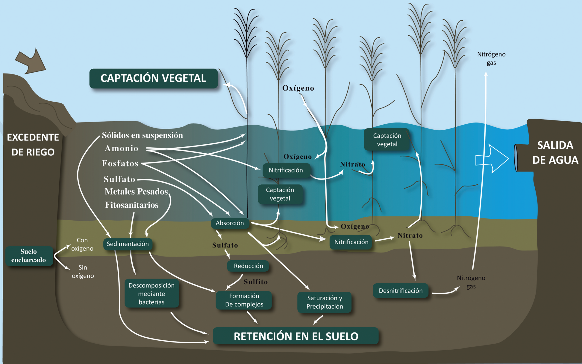
Funcionamiento de un humedal
