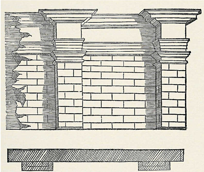
FIG. 10. Disposizione dei pilastri 'a rilievo' in modo che sporgano dalla parete
