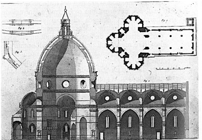
Cupola di Santa Maria del Fiore 1418, 1420-36, Nelli, intercapedine e schema da Sanpaolesi
