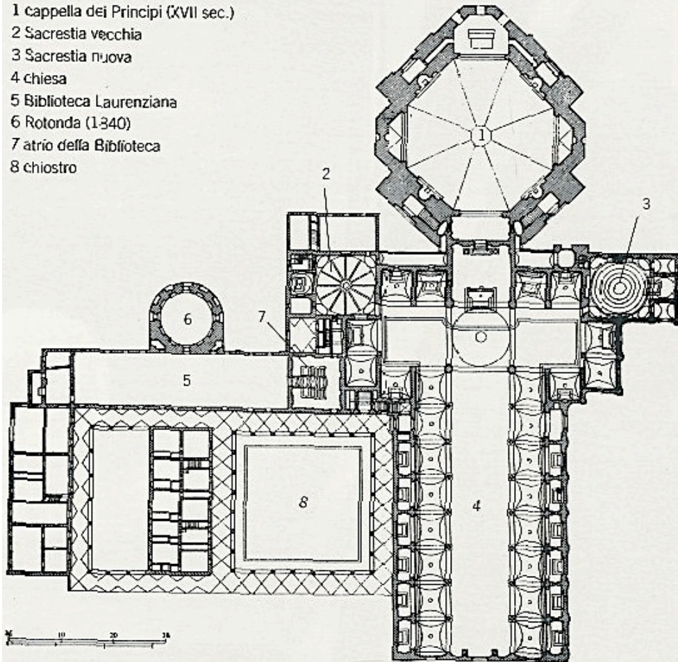
Filippo Brunelleschi, S. Lorenzo, Firenze (iniziata nel 1419): pianta, interno e (in basso a sinistra) veduta della Sacrestia vecchia (1420).
