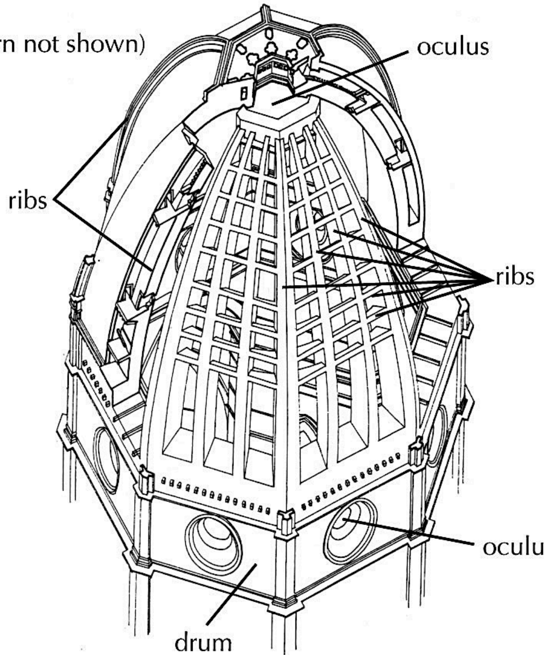
Cupola di Santa Maria del Fiore 1418, 1420-36, Nelli, intercapedine e schema da Sanpaolesi
