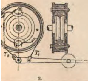
Тормазъ съ кулачками и лентой. 8. Тормазъ автоматическій. 12. Лифтъ гидравлическій. 13, 14, 15. Артиллерійскій подъемъ. Вролгаузъ и Ефронъ, „Энцикл. Слов.“. Сиб., Тип. Ефрона.
