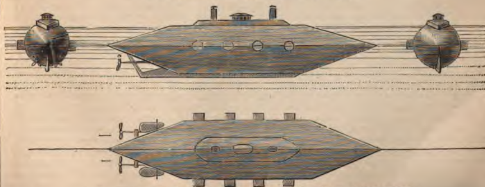
5. Подводная лодка Наутилусъ, строилась въ 1887 въ Вестнидскихъ докахъ.
