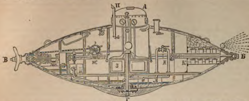
1. Подводный минный аппарат С. К. Девецкаго и подводная лодка „Губа“ въ Шербургѣ, 1887 г.
