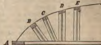
Видъ горизонтальнаго сѣченія набора деревяннаго судна, въ носу. А—фортель; В и С—поворотный шпангоуты; D и E—прямые шпангоуты.
