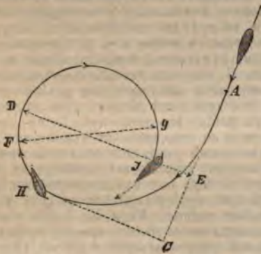
AC—направленіе начальнаго курса судна; A—положеніе судна, когда начали класть руль; длина AC—поступательное перемѣщеніе при поворотѣ; DE—тактический діаметръ; FG—діаметръ циркуляціи; H—положеніе судна, повернувагося на 90°; J—положеніе судна, повернувагося на 360°.
