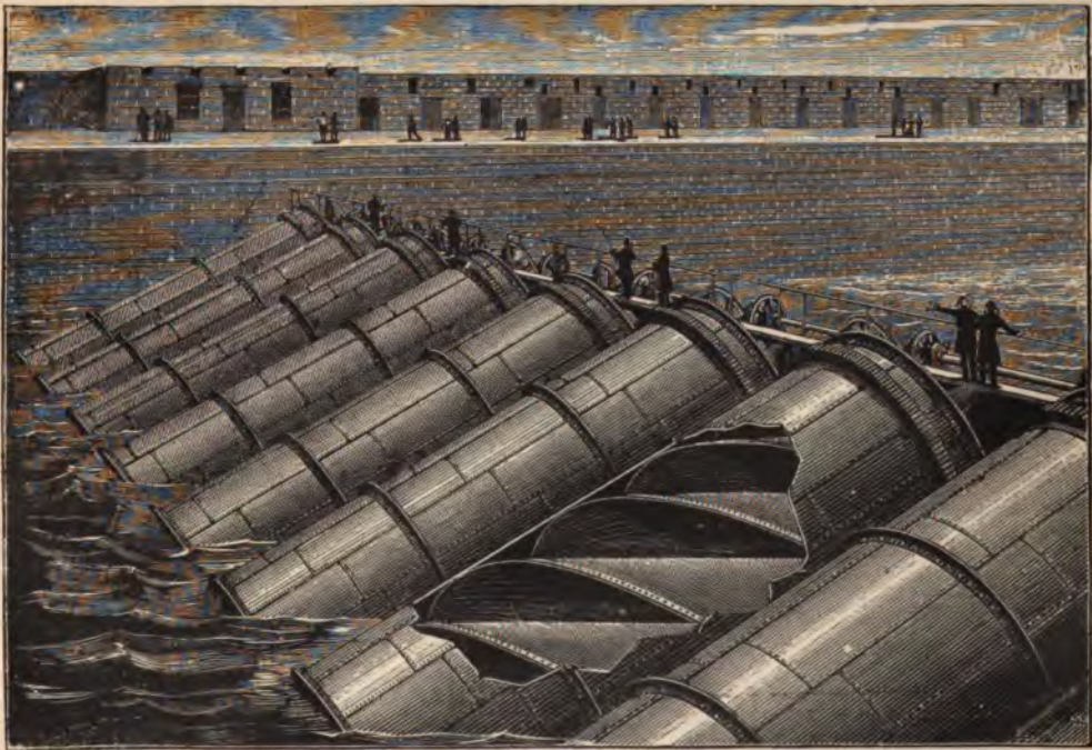
2. Архимедовы винты у г. Катабекъ, на р. Волгѣ.
