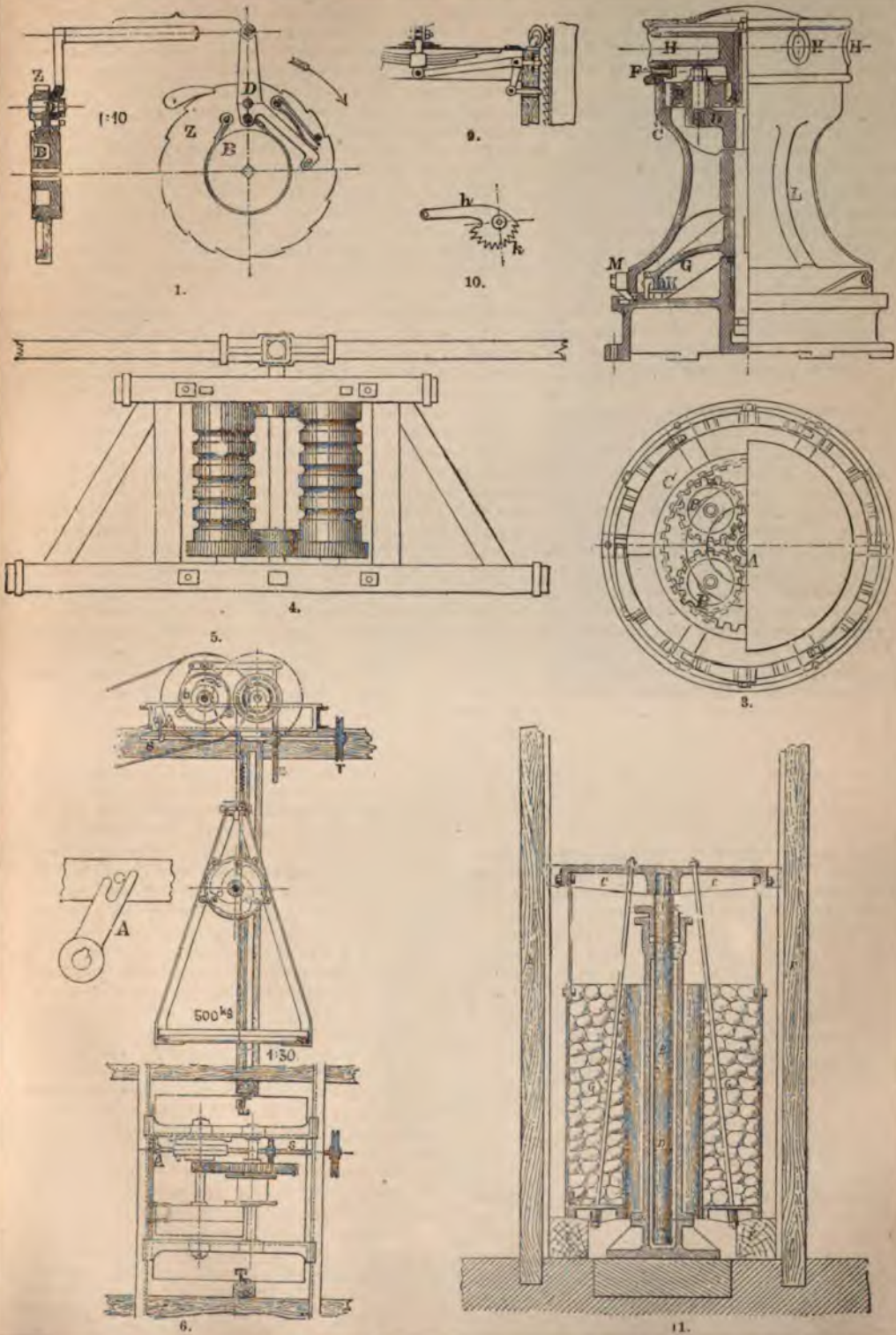
1. Рукоятка не вращающаяся при спуске. 3. Кабестан французский. 4. Лебедка фрикционная. 5. Канатный лифт сбоку. 6. Тоже сверху. 7. Деталь тормазы. 11. Аккумулятор гидравлический. 9 и 10. Парашюты.
