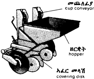
ድንች መትከያ potato planter
