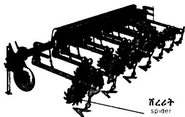
ተሽከርካሪ መጎተቻ rotary hoe
