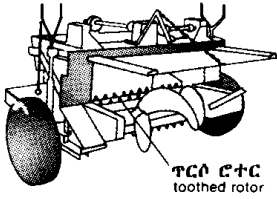
ትሪት መበተኛ field heap spreader
