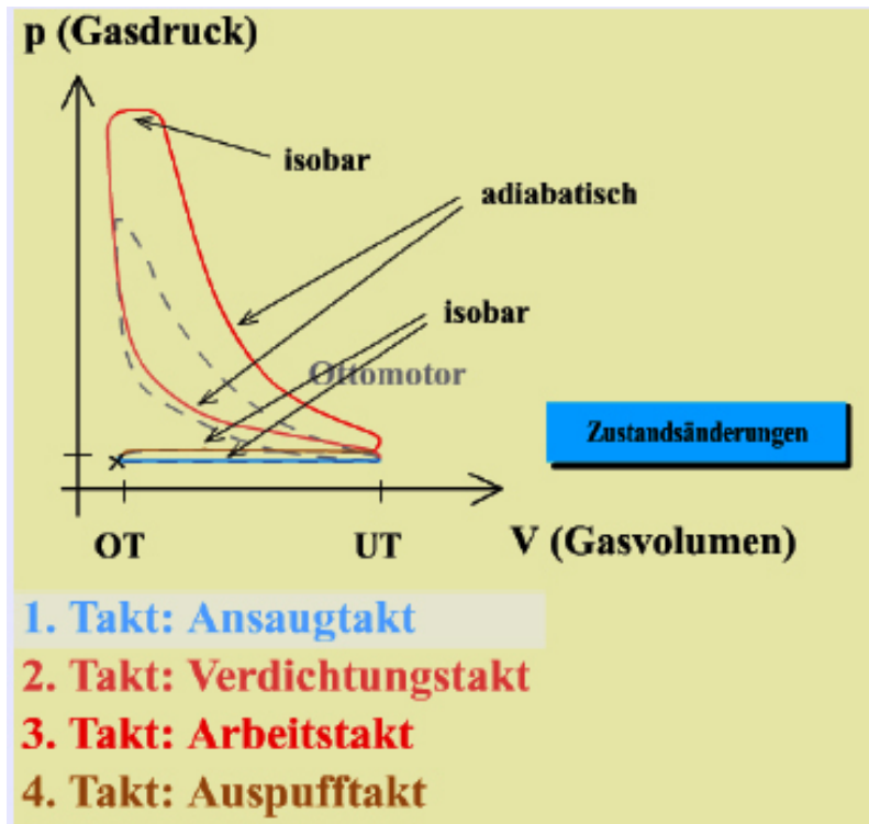
Abb. 8: Zustandsänderungen beim Dieselmotor
