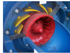
Abb. 17: Leitwerk einer Francis-Turbine für maximale Leistung eingestellt
