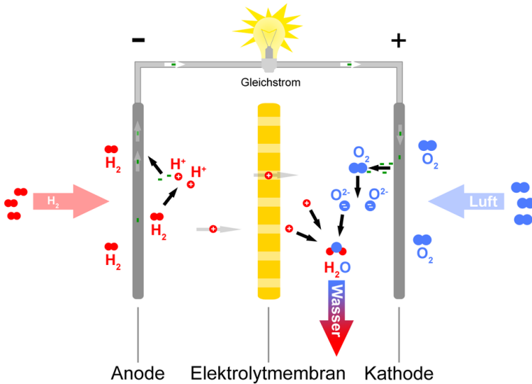
Abb. 19: Funktionsprinzip einer Brennstoffzelle
