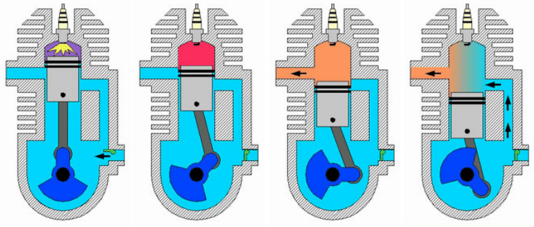
Abb. 6: Vorgänge des 2. Taktes oberhalb und unterhalb des Zylinderkolbens (Schritt für Schritt von links nach rechts)
