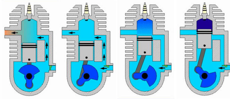
Abb. 5: Vorgänge des 1. Taktes oberhalb und unterhalb des Zylinderkolbens (Schritt für Schritt von links nach rechts)
