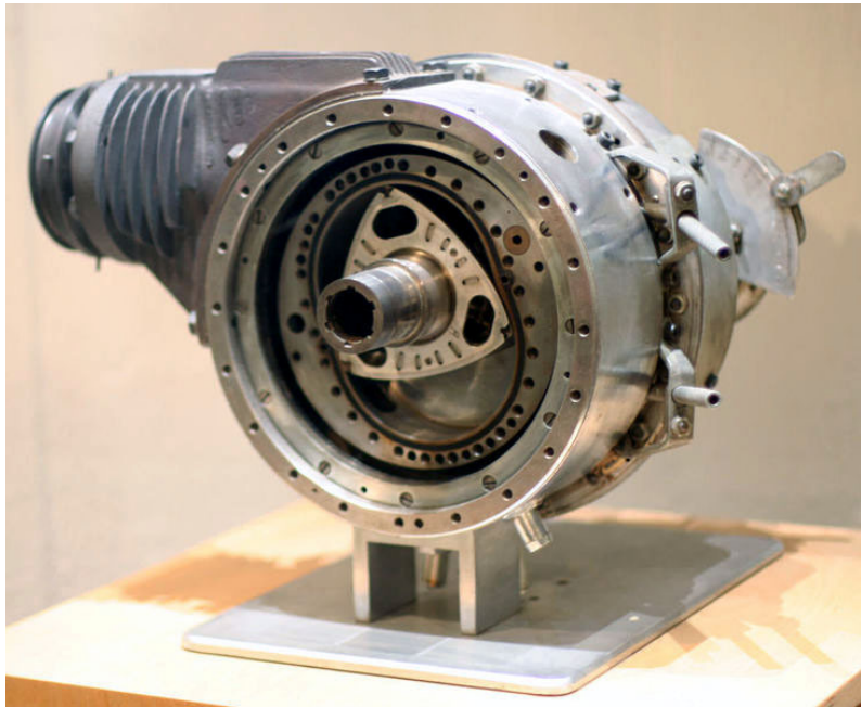
Abb. 9: Felix Wankels Drehkolbenmotor DKM 54
