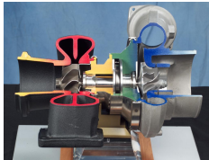
Abb. 15: Querschnitt eines Abgasturboladers
