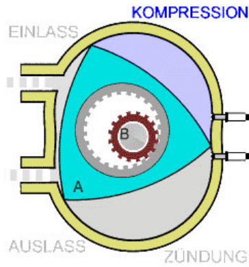
Abb. 11: 2. Takt: Kompression / Verdichten
