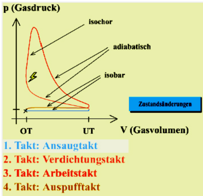
Abb. 7: Zustandsänderungen beim Ottomotor
