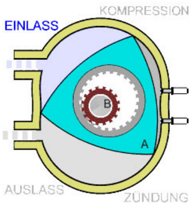
Abb. 10: 1. Takt: Einlass / Ansaugen
