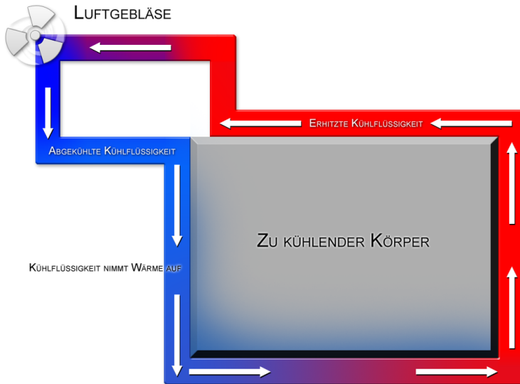
Abb. 18: Funktionsprinzip einer einfachen Flüssigkeitskühlung
