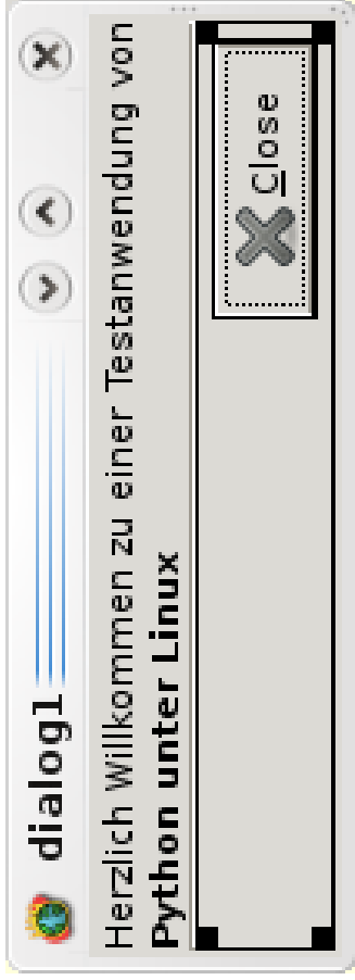
Abb. 16 Der Dialog
