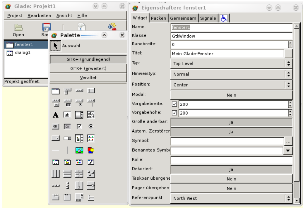
Abbildung 14: Benutzeroberfläche in Glade erstellen
