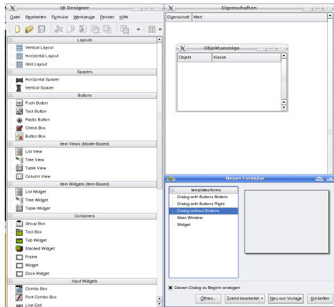
Abbildung 10: Designer
