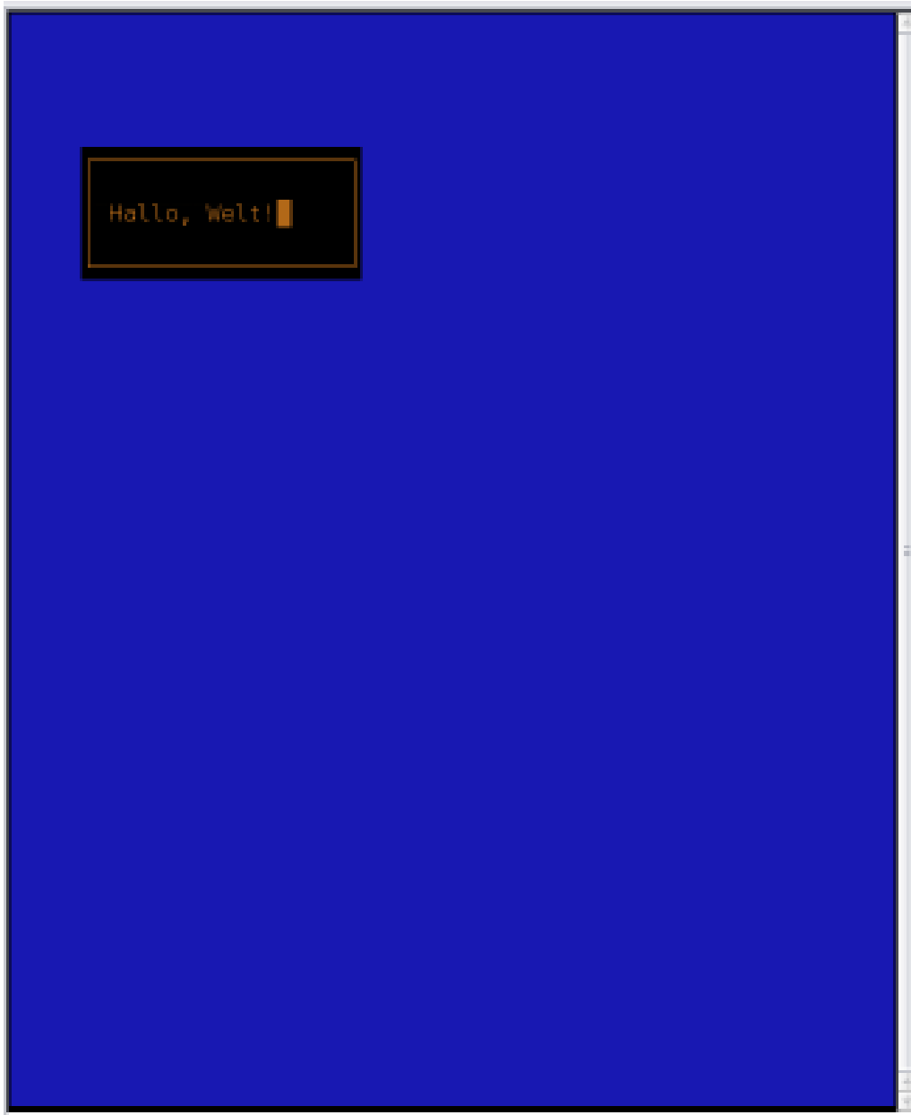
Abbildung 17: Hallo Welt
