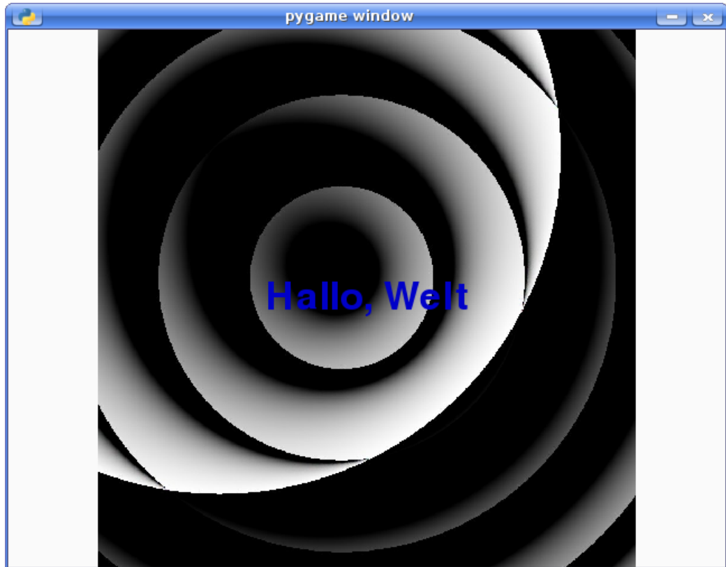
Abbildung 5: Bilder anzeigen
