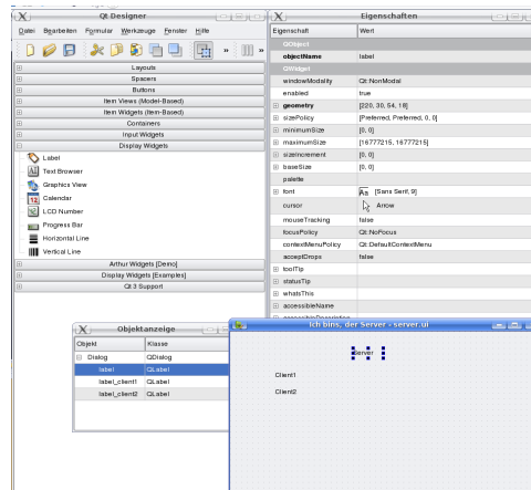
Abbildung 11: Unser Dialogfenster
