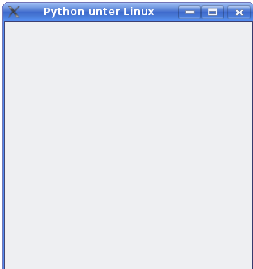
Abbildung 6: guiqt1.py
