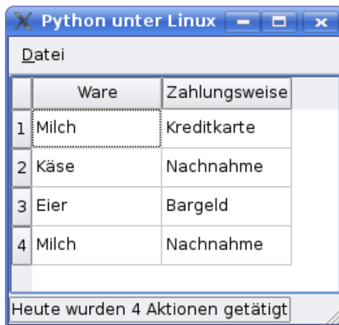
Abbildung 8: guiqt3.py Anwendung
