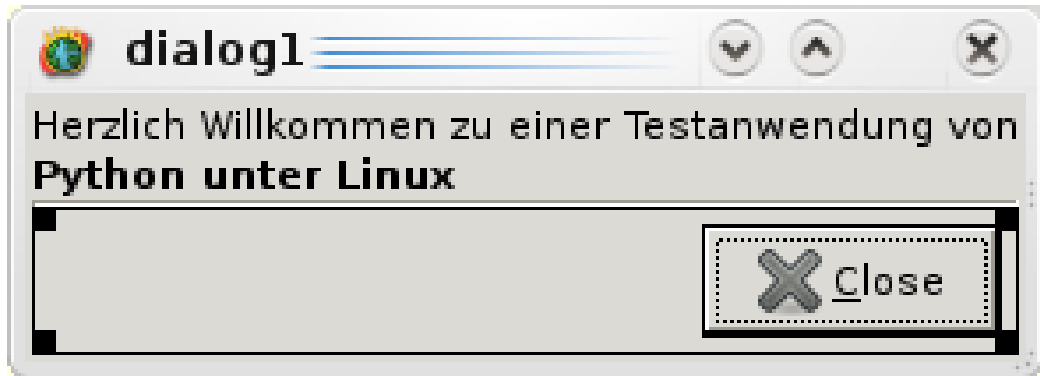
Abbildung 16: Der Dialog
