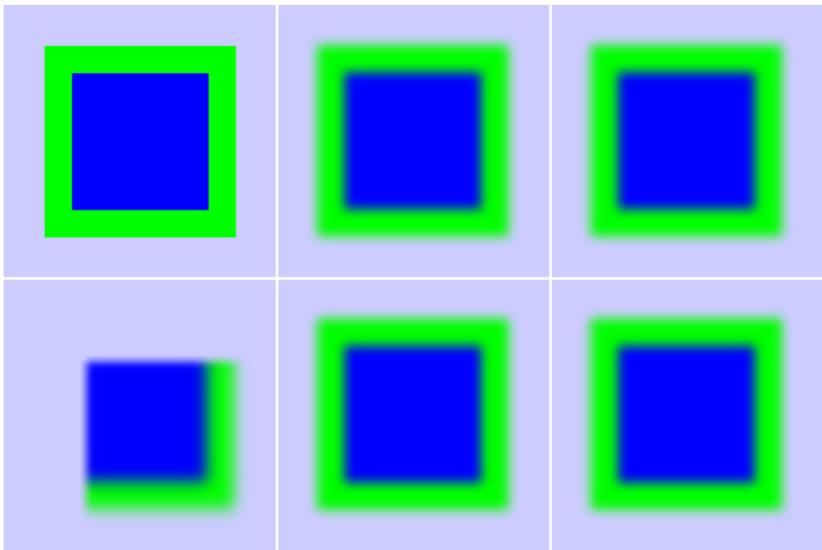
Abb. 310 filter -Beispiele
