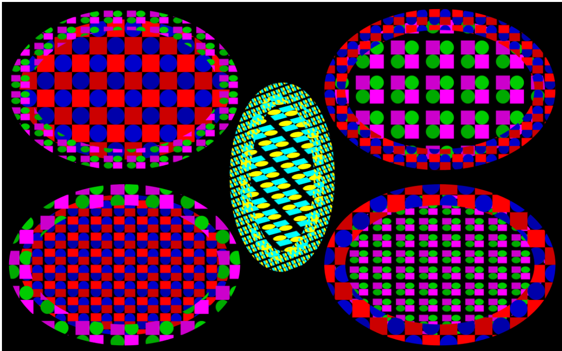
Abb. 178 einige Muster
