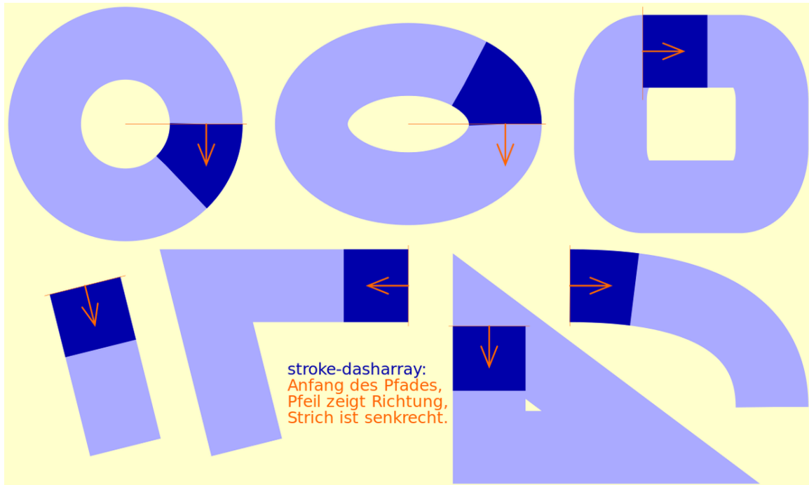
Abb. 116 Beispiel (2) stroke-dasharray
