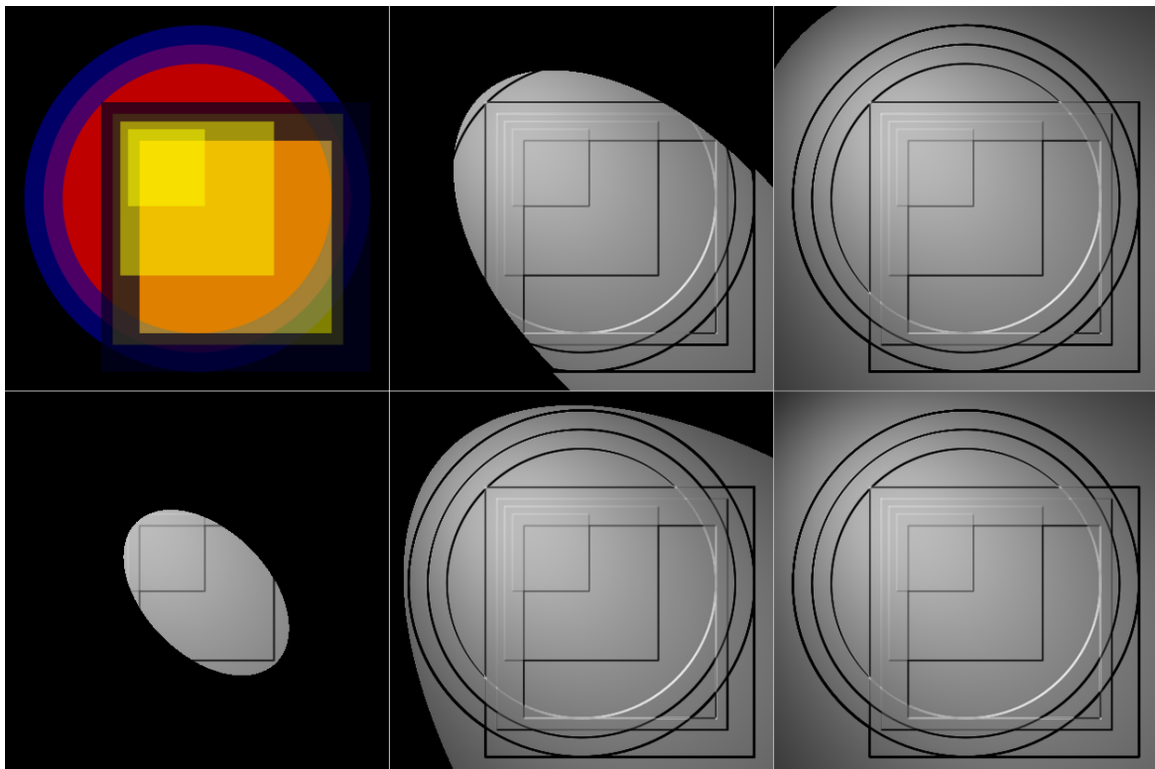
Abb. 373 Strahlkegel
