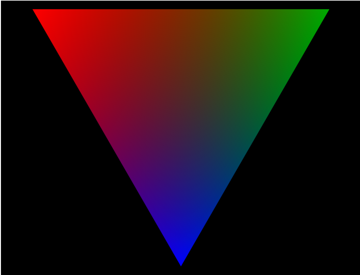
Abb. 171 Farbverlaufsdreieck
