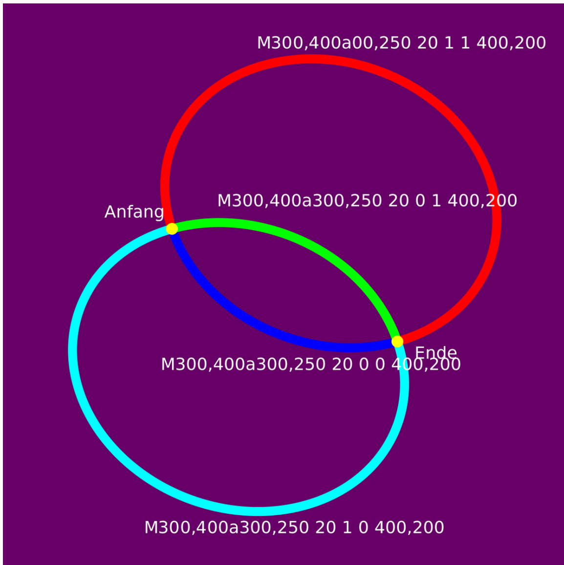
Abb. 84 Pfadkommando a
