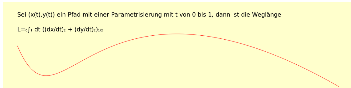
Abb. 299 Weglänge
