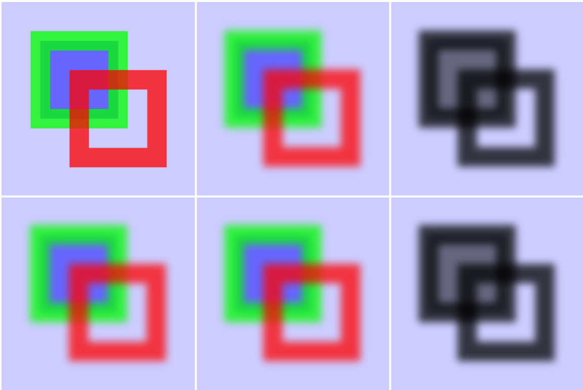
Abb. 312 Eingabemöglichkeiten (2)
