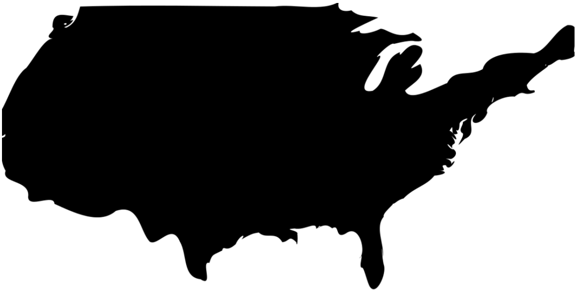
Abb. 210 Pfad
