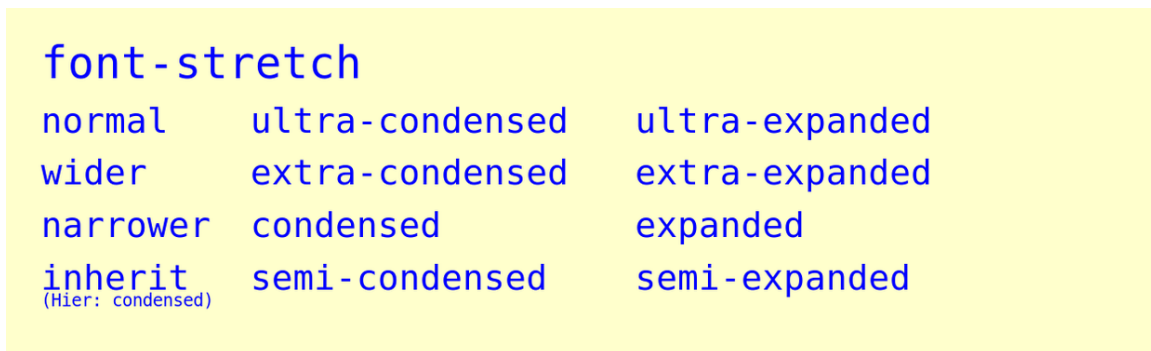
Abb. 133 Beispiel Schriftdehnung
