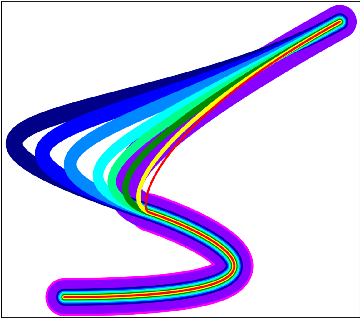
Abb. 79 Fortsetzungen eines kubischen Pfades ohne Knicke, Kommando s
