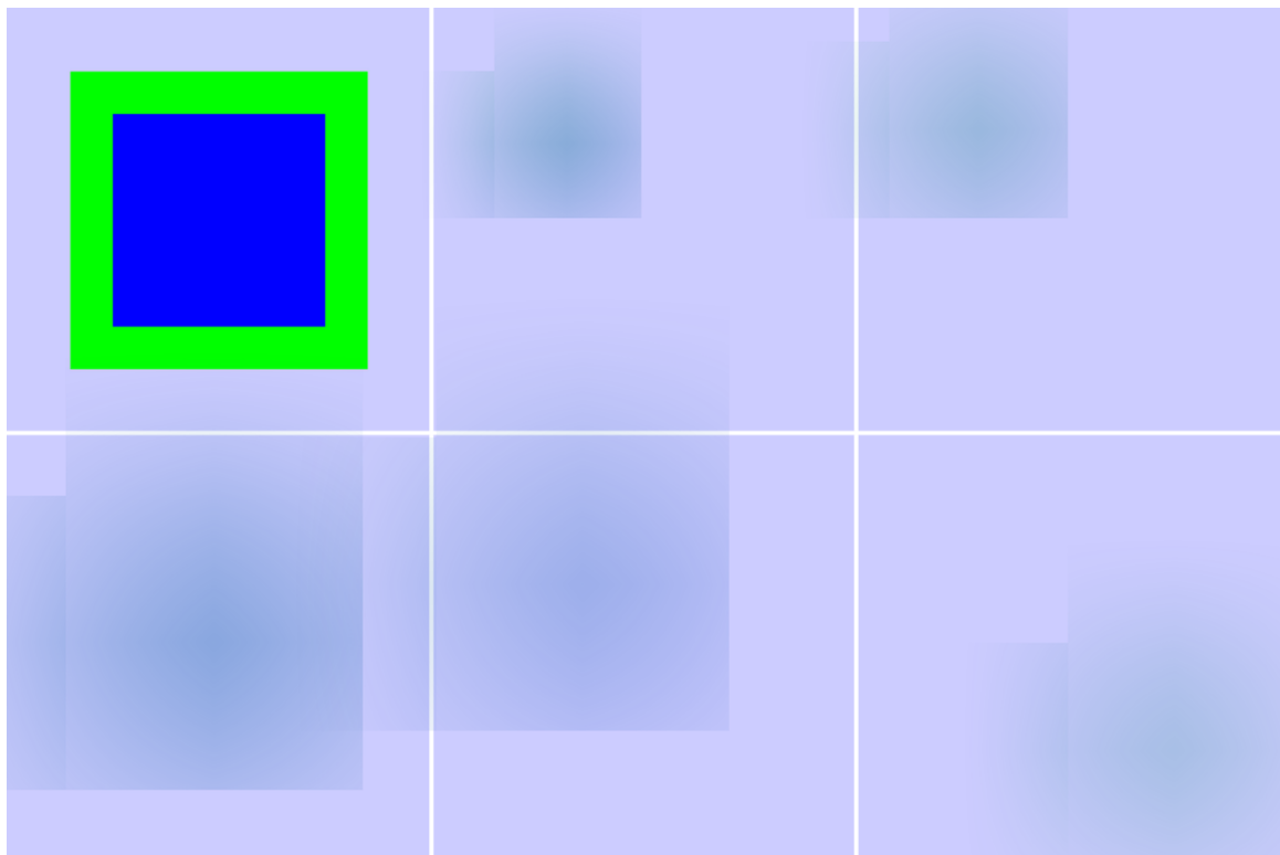
Abb. 306 relative Koordinaten (1)
