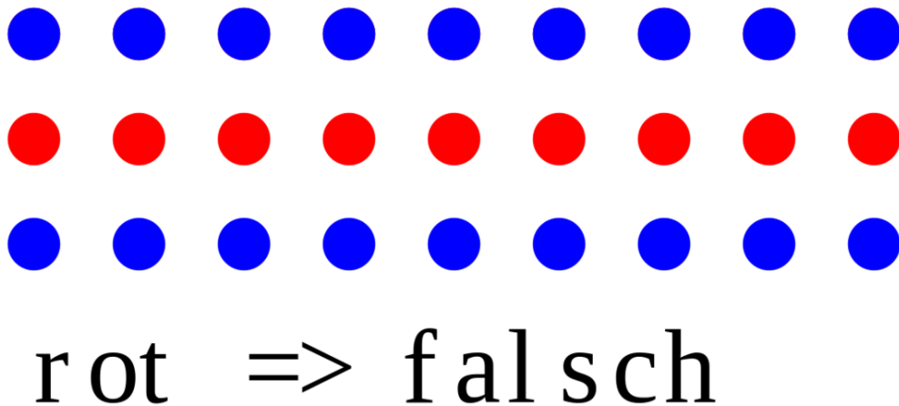
Abb. 69 Pfade der Länge 0
