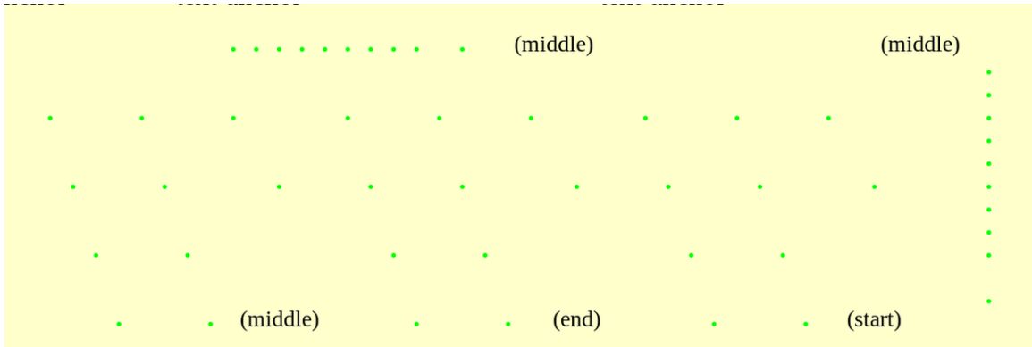
Abb. 140 Beispiel text-anchor (2)
