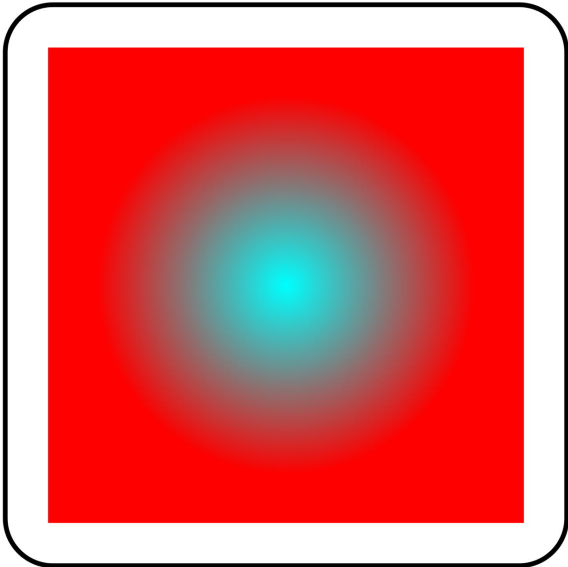
Abb. 162 radialGradient
