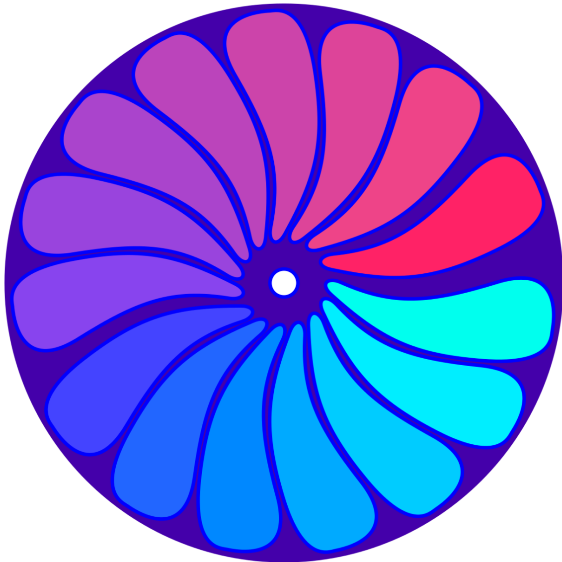
Abb. 289 Einfaches Musikinstrument
