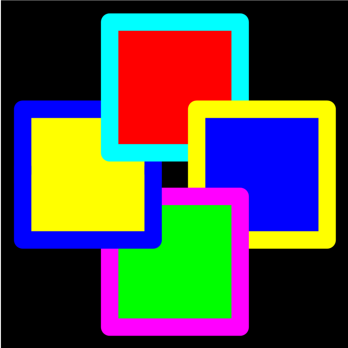
Abb. 13 Verkeilte Vierecke
