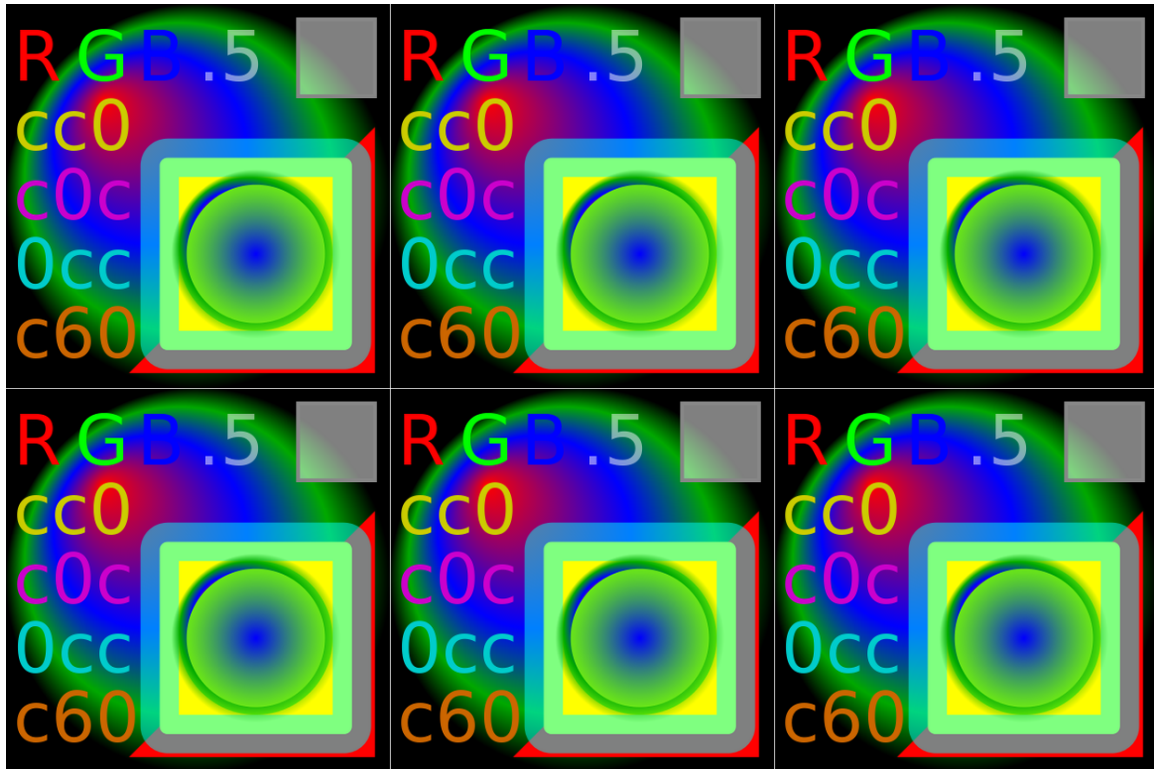
Abb. 339 nach Tabelle
