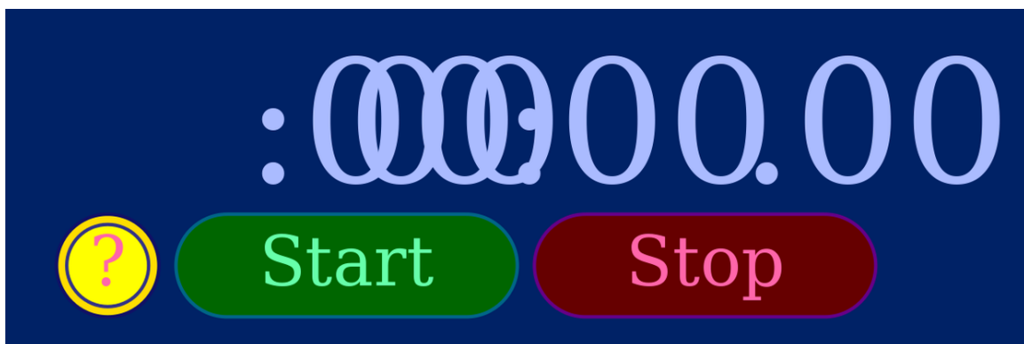
Abb. 268 Digitale Stopuhr
