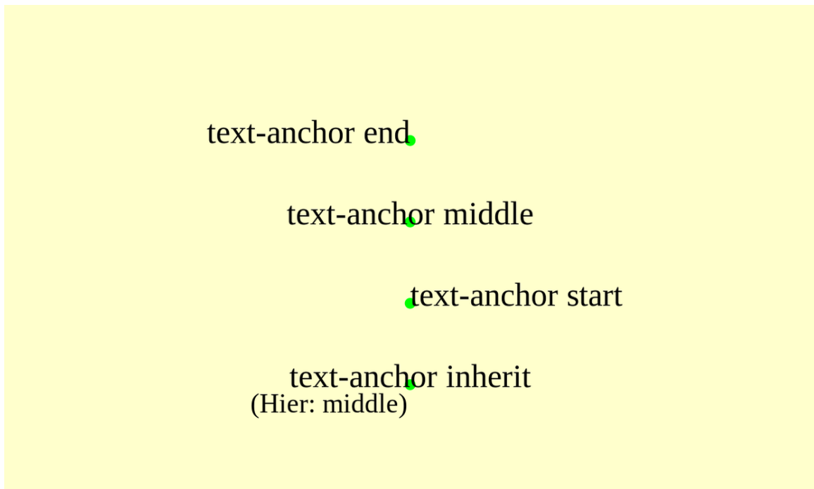
Abb. 139 Beispiel text-anchor
