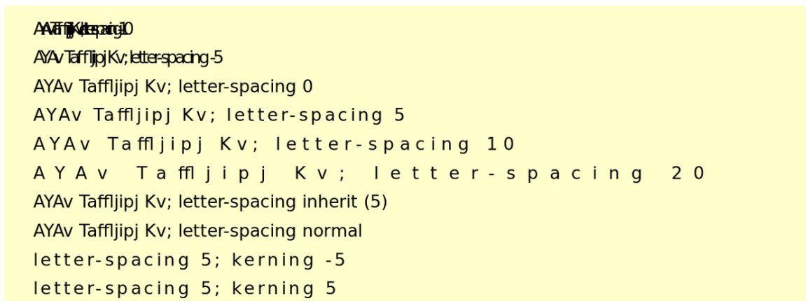
Abb. 147 Beispiel letter-spacing
