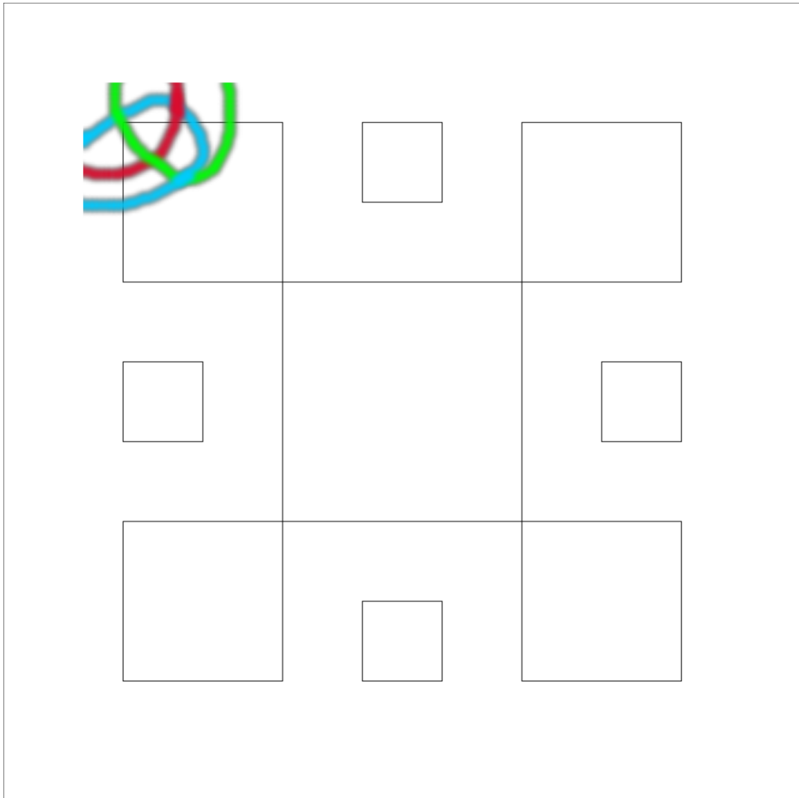
Abb. 325 Bilder einbetten (1)
