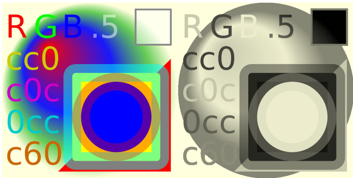
Abb. 333 Leuchtdichte
