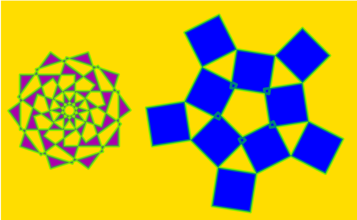
Abb. 73 Spielerei mit Unterpfaden, bestehend aus Quadraten - Beispiel für Kommandos 'L' und 'l'
