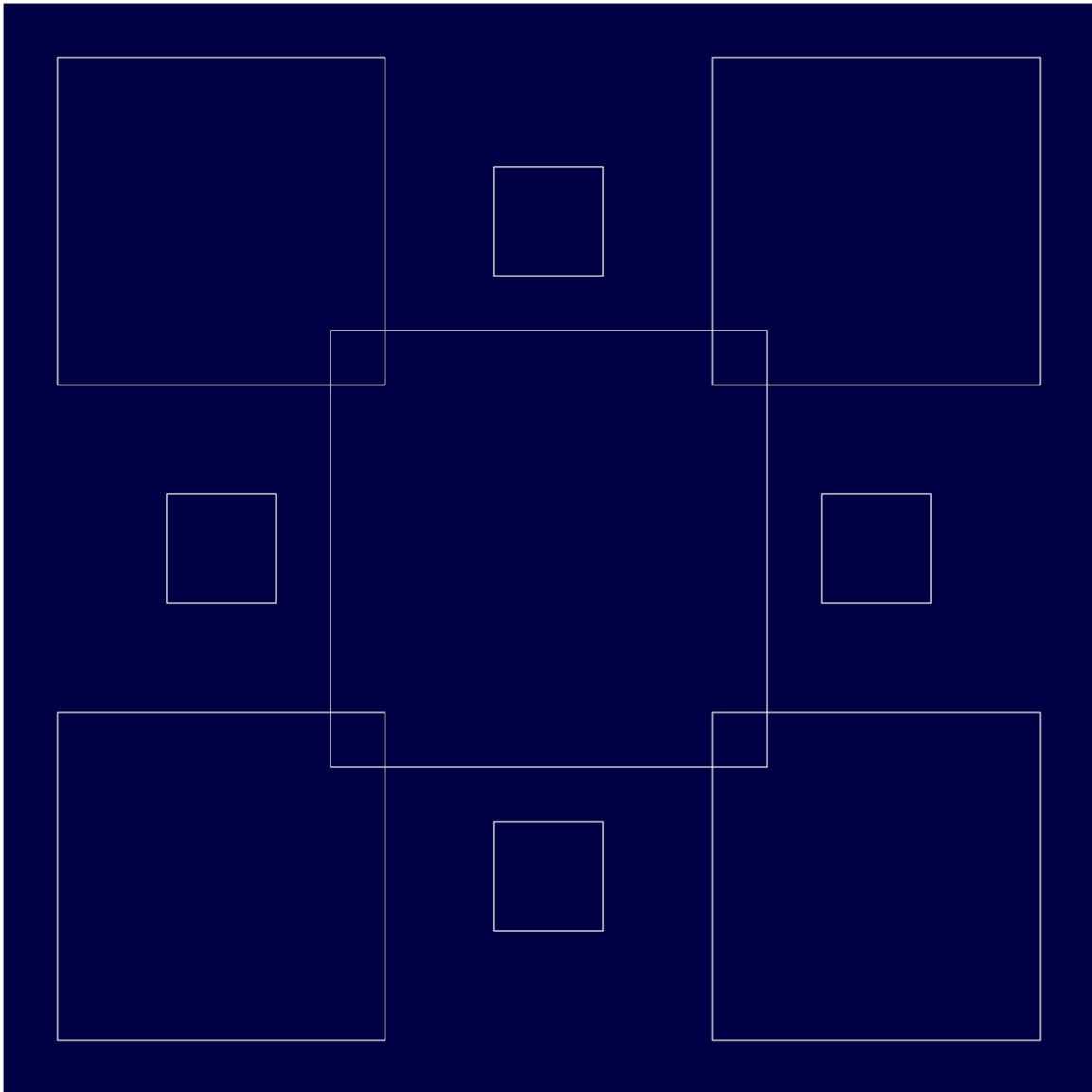
Abb. 328 Zusammenfügen
