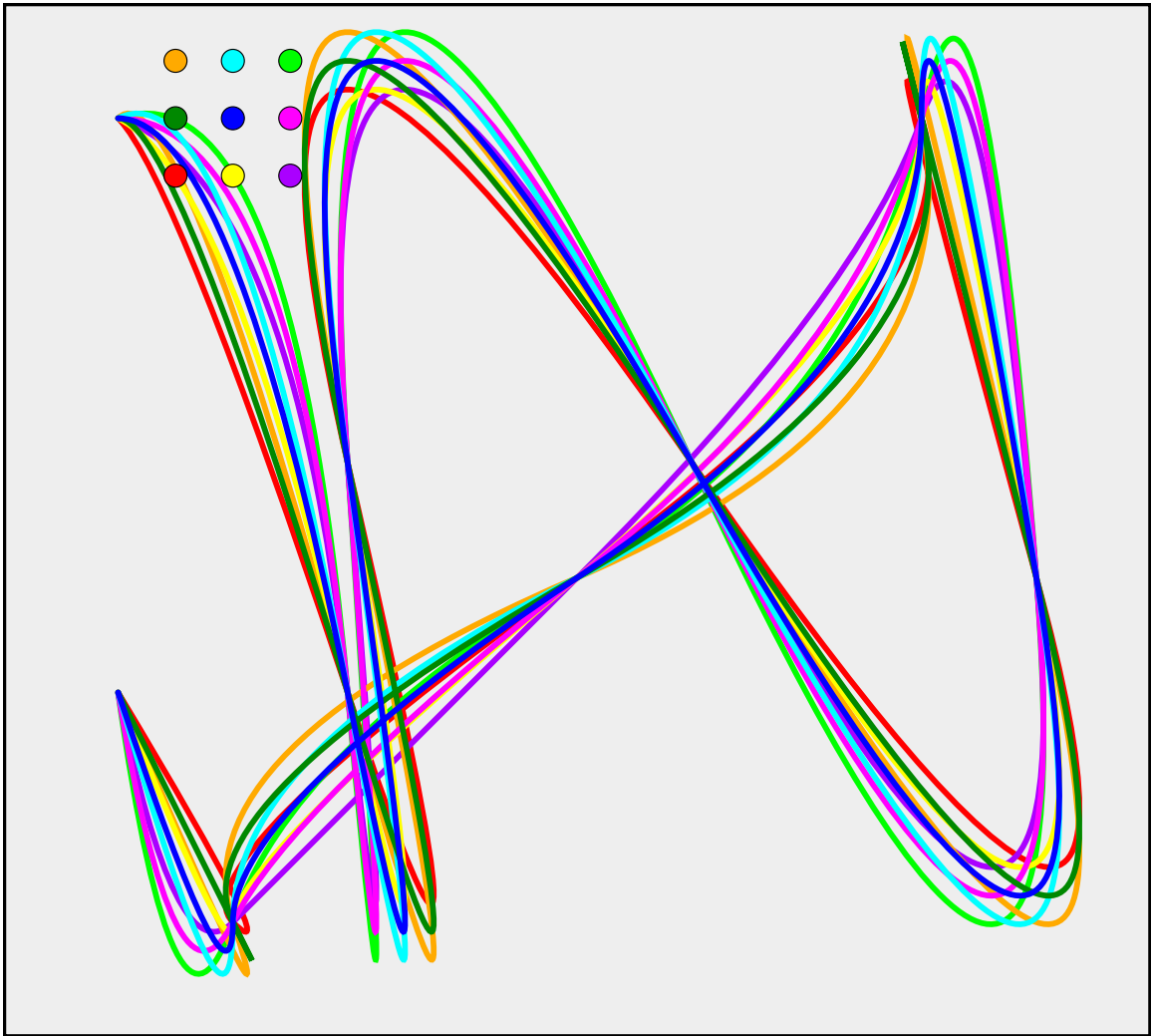
Abb. 73 Nichtlokalität von Kontrollpunkten in QT-Pfaden
