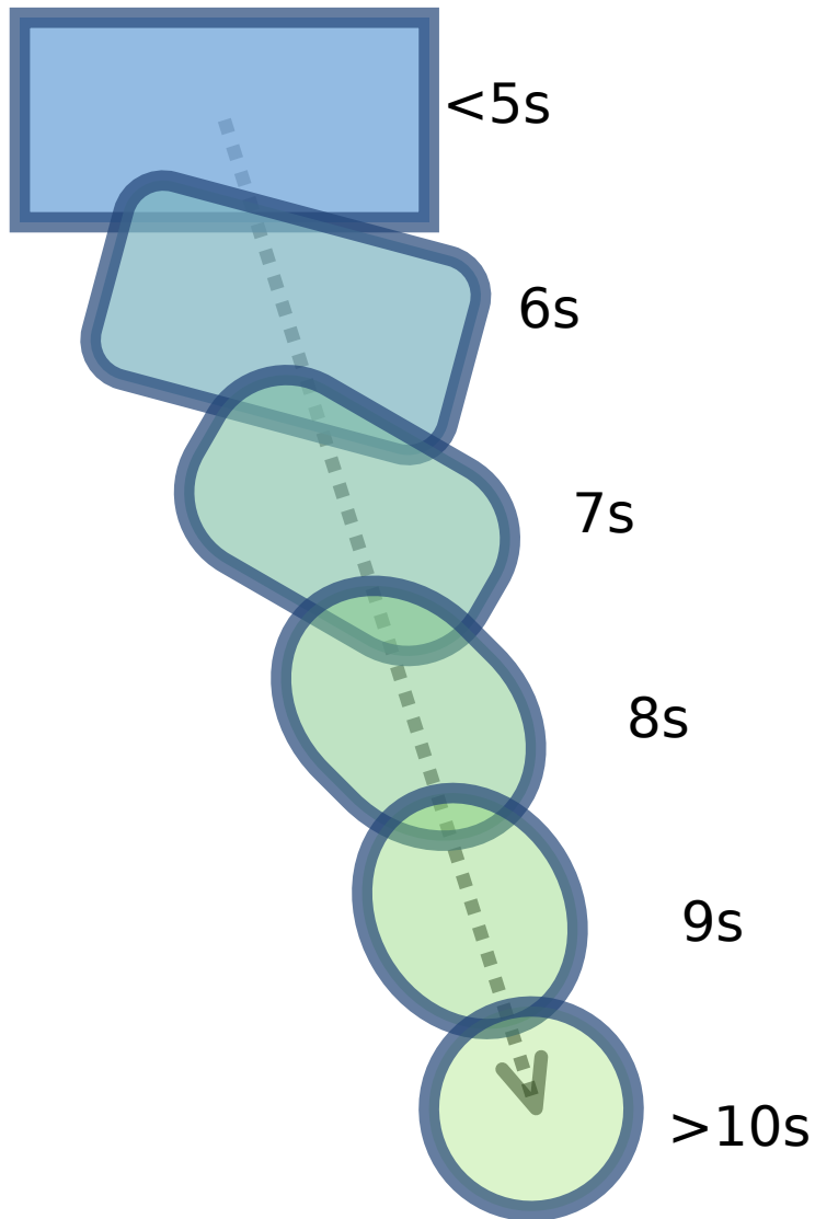
Abb. 98 BEISPIEL UND SCHEMATISCHE DARSTELLUNG EINER ANIMATION IN SVG a : Gleichzeitige Animation von Breite, Radius der abgerundeten Ecken, Position, Füllfarbe und Füllopazität eines Rechteckes über 5 Sekunden.
