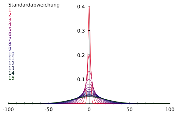
Abb. 115 Gaußkurven mit verschiedenen Standardabweichungen
