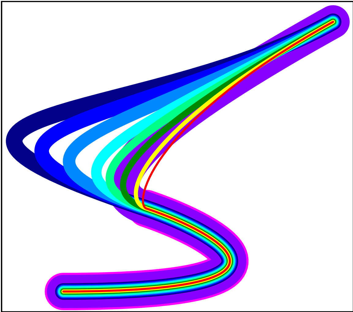
Abb. 76 Fortsetzungen eines kubischen Pfades ohne Knicke, Kommando s
