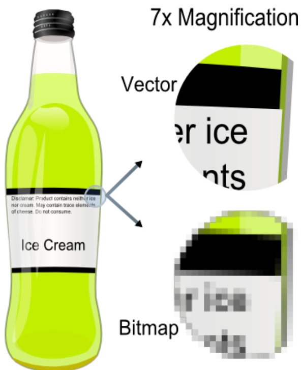
Abb. 1: Vektorgrafiken lassen sich ohne Qualitätsverlust beliebig skalieren.
