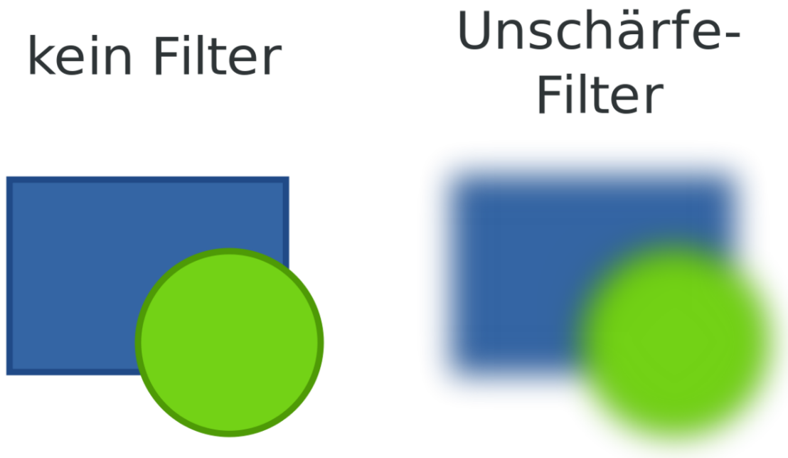
Abb. 44: Quellgraphik und Ergebnis eines Gaußfilters
