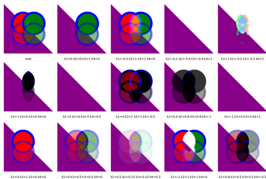
Abb. 64: Kompositionen, arithmetischer Operator
