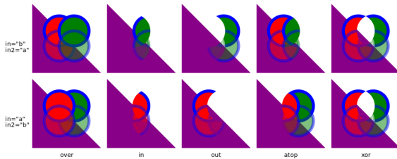
Abb. 63: Kompositionen, einfache Operatoren
