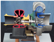
Abb. 15: Querschnitt eines Abgasturboladers
