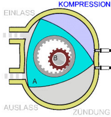
Abb. 11: 2. Takt: Kompression / Verdichten
