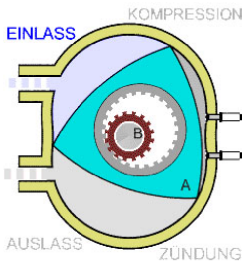
Abbildung 10: 1. Takt: Einlass / Ansaugen
