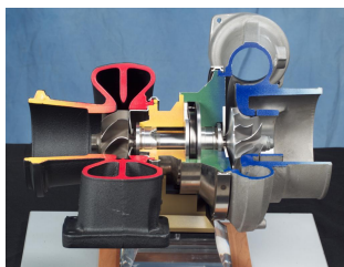
Abbildung 15: Querschnitt eines Abgasturboladers
