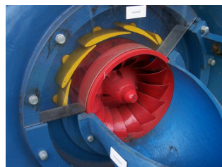
Abbildung 16: Leitwerk einer Francis-Turbine für minimale Leistung eingestellt
