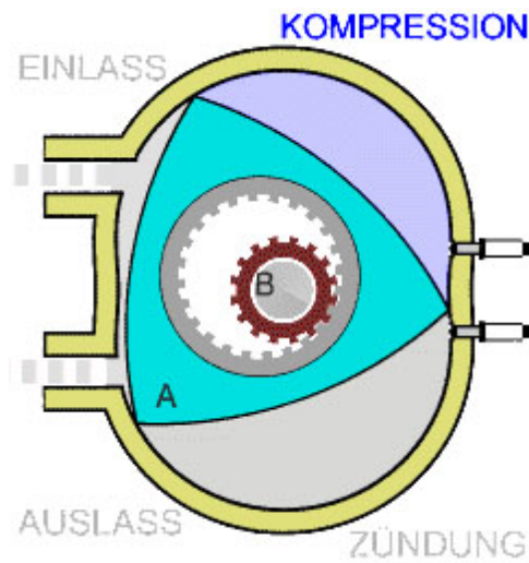
Abbildung 11: 2. Takt: Kompression / Verdichten
