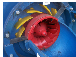
Abbildung 17: Leitwerk einer Francis-Turbine für maximale Leistung eingestellt
