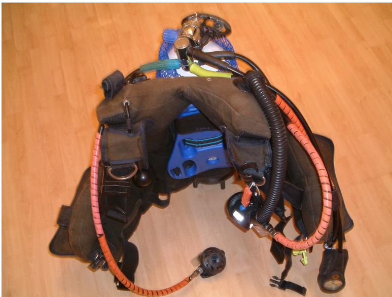
Abbildung 56: Vollständiges Drucklufttauchgerät mit Druckluftbehälter, Lungenautomat (hier Octopussystem), optischer Reserwarneinrichtung und Jacket (Kombination aus Rettungs- und Tariermittel und Tragevorrichtung)
