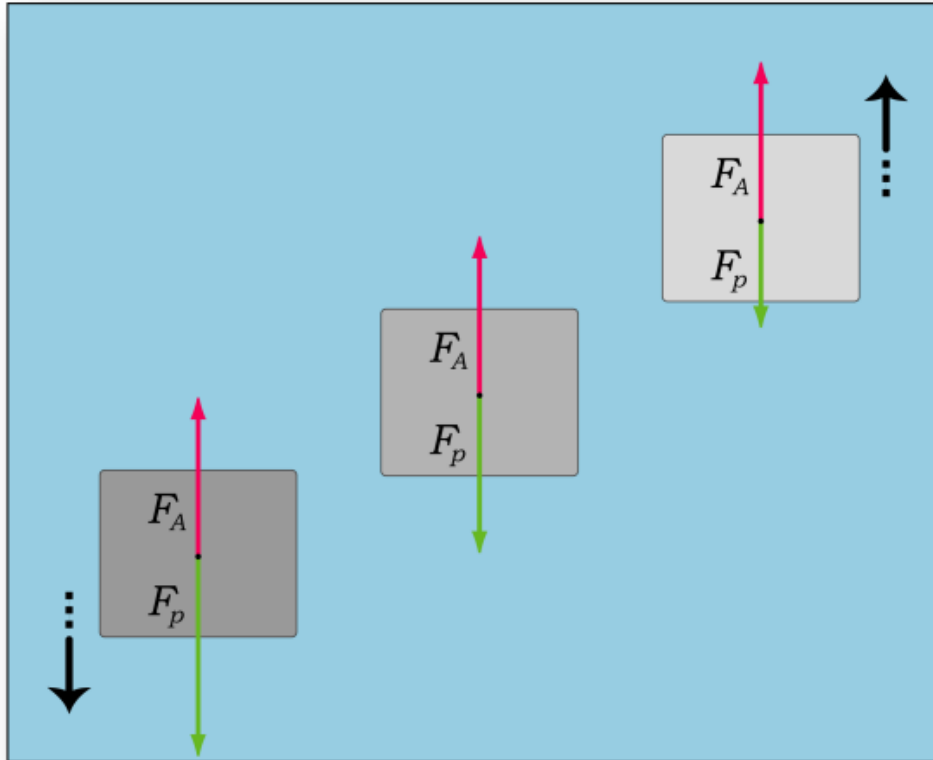
Abbildung 18: Hydrostatische Zustände eines Körpers: Schwimmen, Schweben, Sinken
