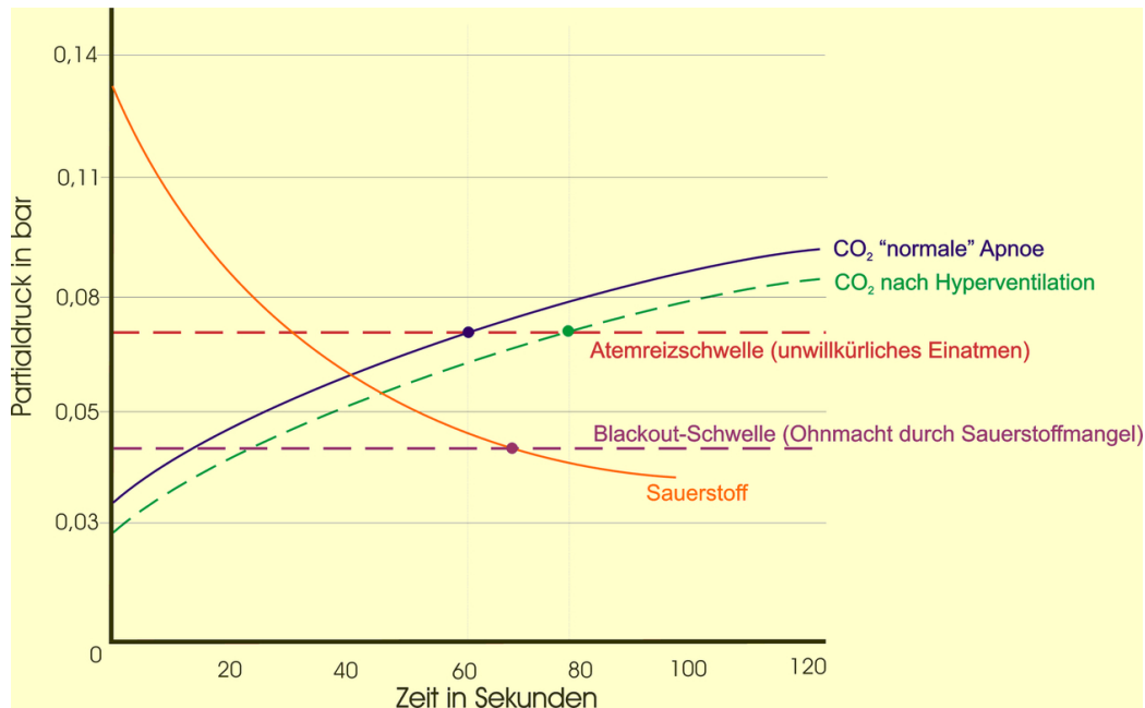
Abbildung 40: Nach dem Hyperventilieren wird die kritische Black-Out-Schwelle des Sauerstoffs unterschritten bevor der CO 2 -Partialdruck die Atemreizschwelle erreicht
