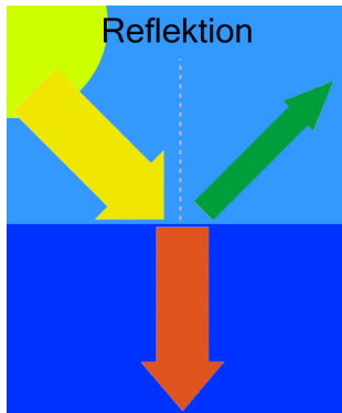
Abbildung 19: Die Reflexion an der Wasseroberfläche vermindert die Quantität des Lichtes unter Wasser.
