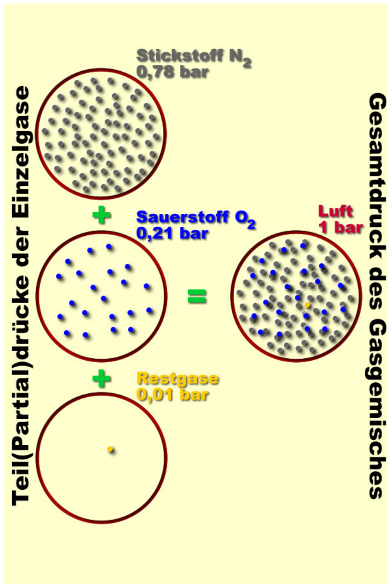
Abbildung 16: Gesetz von Dalton: Der Gesamtdruck eines Gasgemisches, ist gleich der Summe der Teildrücke, der in ihm enthaltenen Partialgase.
