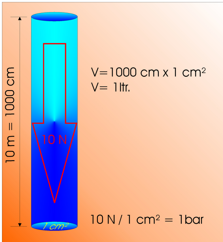
Abbildung 10: Eine Wassersäule von 10m Höhe erzeugt einen Druck von einem Bar
