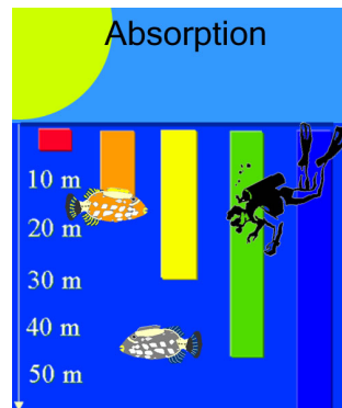
Abbildung 23: Mit zunehmenden Weg des Lichtes durch das Wasser werden die Spektralanteile des weißen Lichtes absorbiert. Gegenstände "verlieren" mit zunehmender Entfernung und Tiefe ihre Farben, die dann "Grau" erscheinen.
