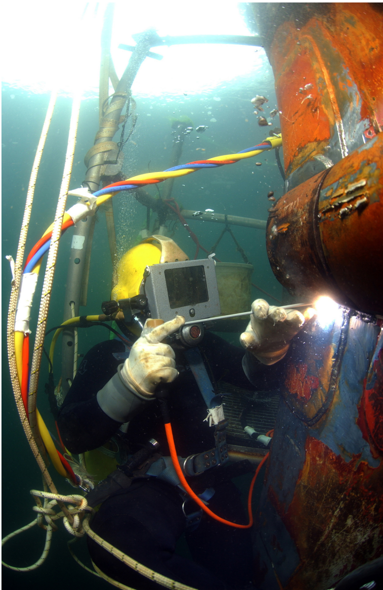
Abbildung 46: Helmtaucher bei Unterwasserarbeiten
