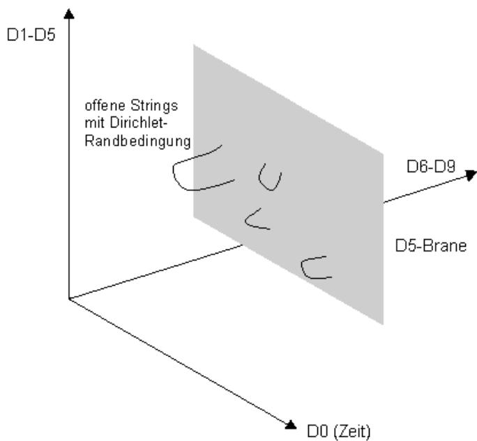
Abb. 25: D-Brane mit Strings, die der Dirichlet-Randbedingung genügen
