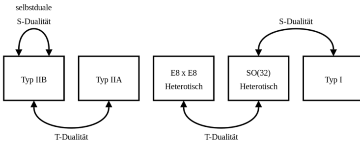
Abb. 20: Dualitäten zwischen den Stringtheorien
