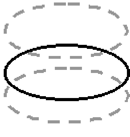
Schwerpunktschwingung
