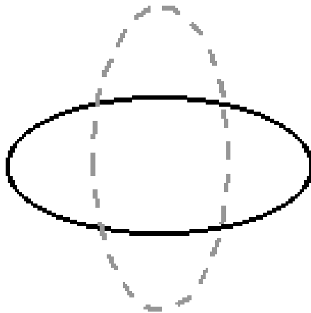
Schwingung
