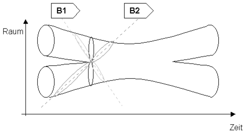
Wechselwirkung von Strings aus der Sicht zweier sich in Relativbewegung zueinander befindenden Beobachter
