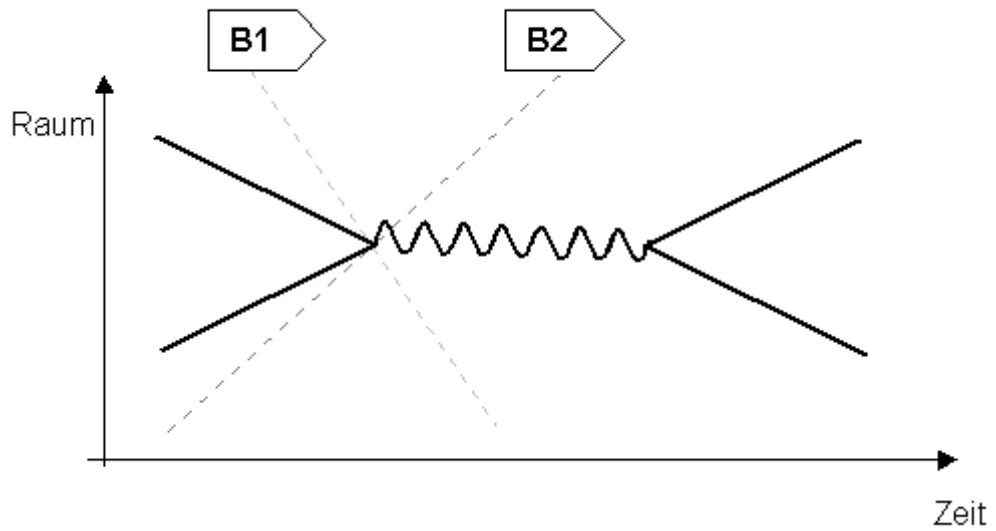
Feynman Diagramm: Wechselwirkung von Punktteilchen aus der Sicht zweier sich in Relativbewegung zueinander befindenden Beobachter
