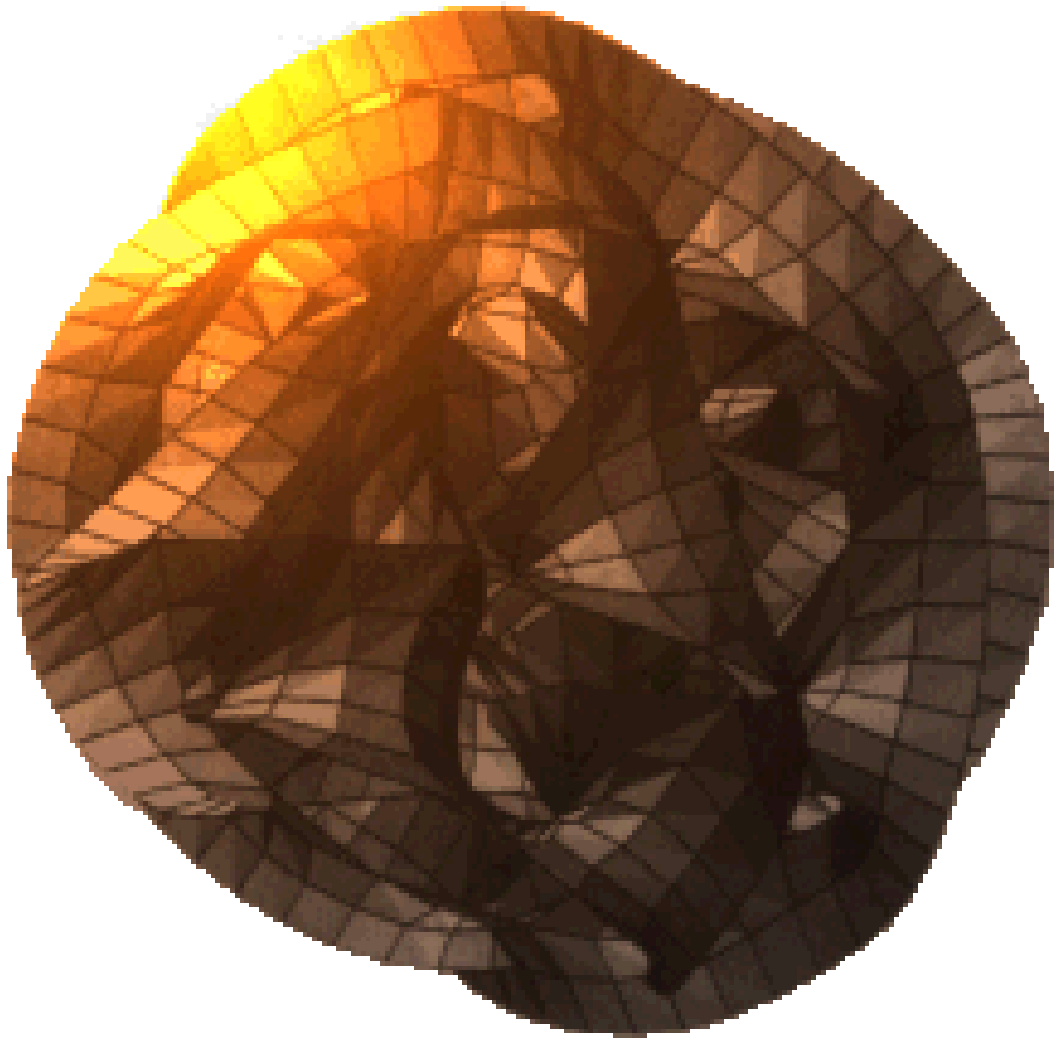
Calabi-Yau-Mannigfaltigkeit
