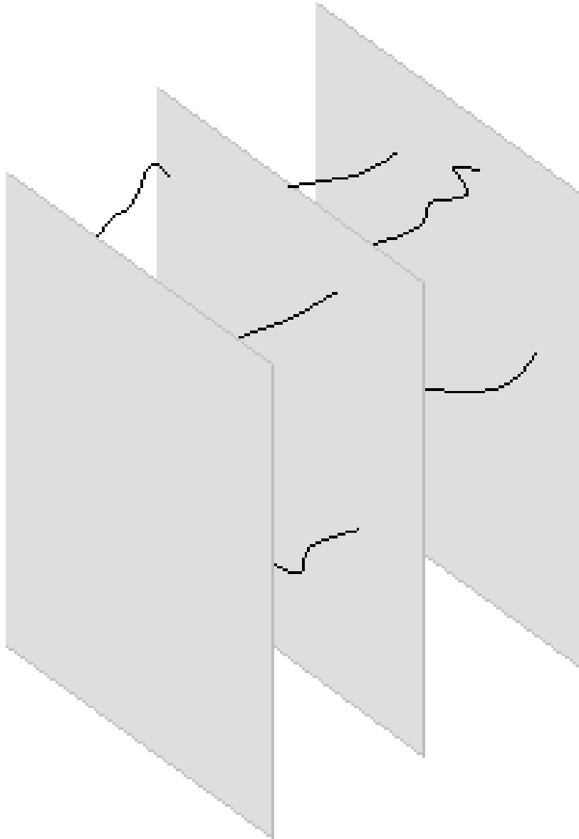
Strings zwischen D-Branen
