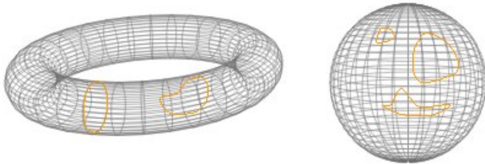
Strings auf der Oberfläche einer Kugel oder eines Torus
