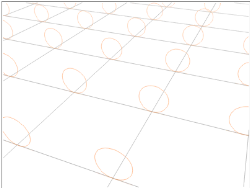
Eine aufgewickelte Dimension an jedem Punkt der Raumzeit
