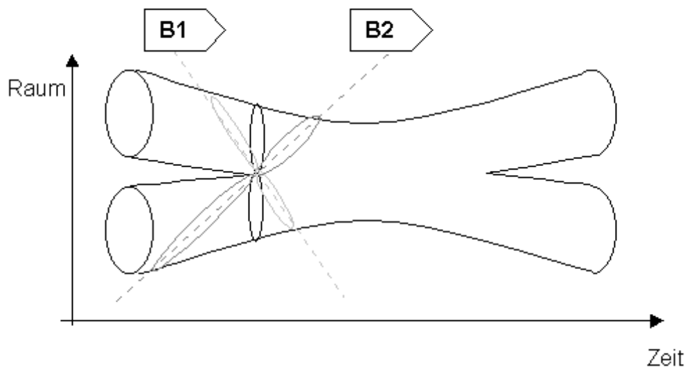
Wechselwirkung von Strings aus der Sicht zweier sich in Relativbewegung zueinander befindenden Beobachter
