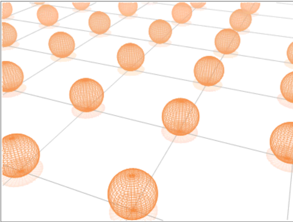
Zwei Dimensionen zu einer Kugel aufgerollt
