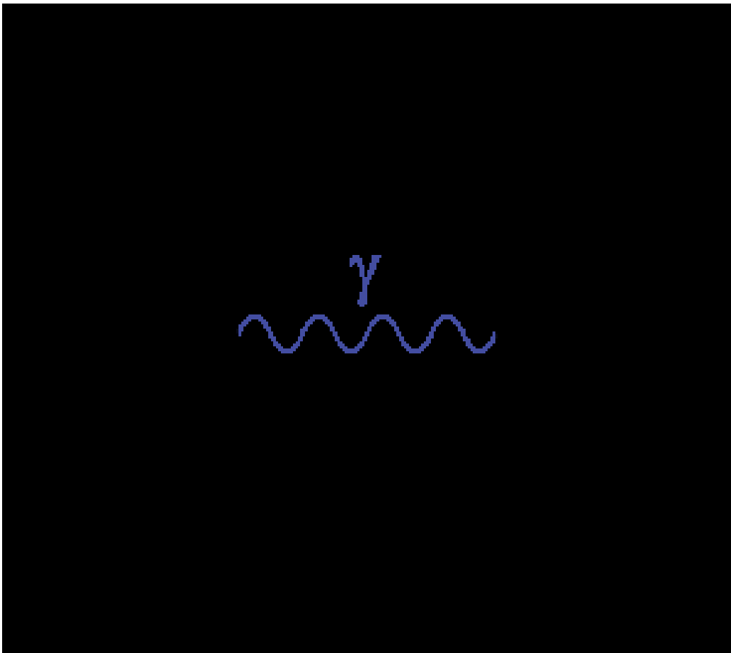
Punktteilchenwechselwirkung von Elektron und Positron
