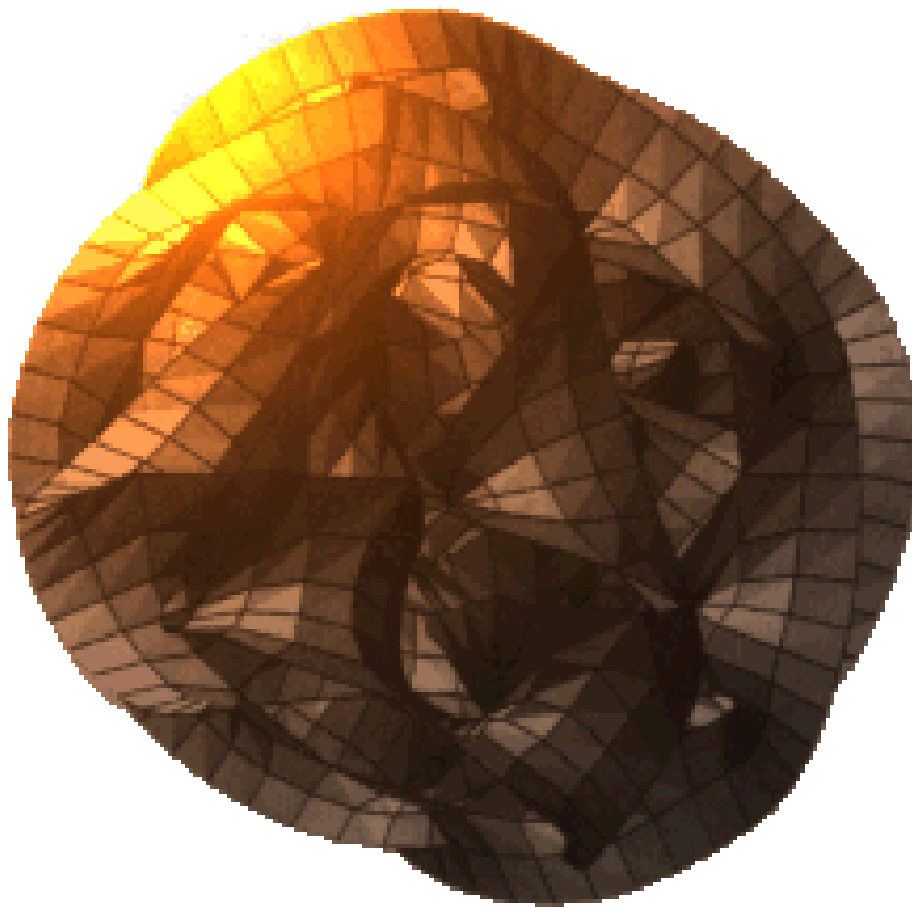
Strings auf der Oberfläche einer Kugel oder eines Torus
