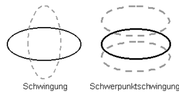
Abbildung 3.1: Schwerpunktschwingung eines Strings
