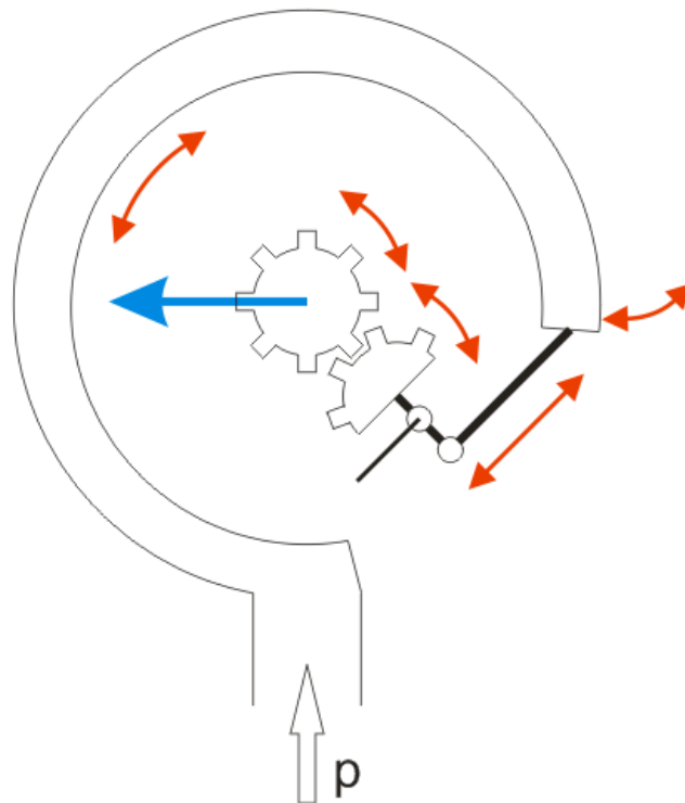
Abbildung 54: Wirkschema eines UW-Manometers mit Rohrfeder-Prinzip
