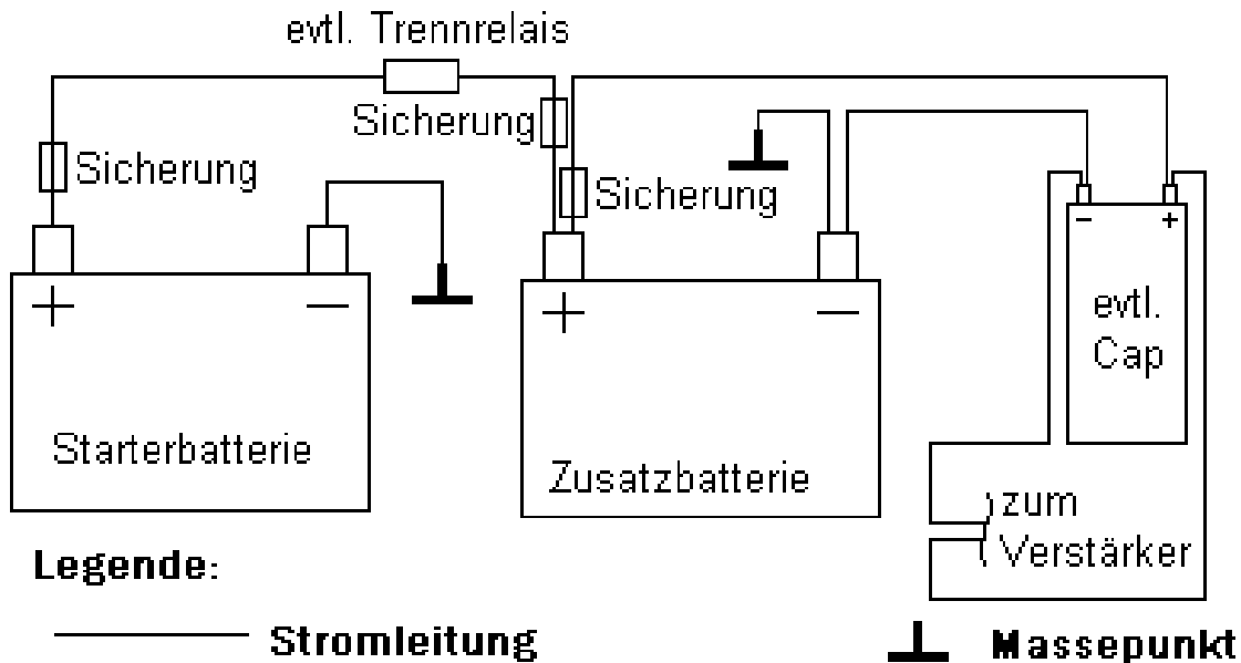
Abb. 3 Schematische Verschaltung
