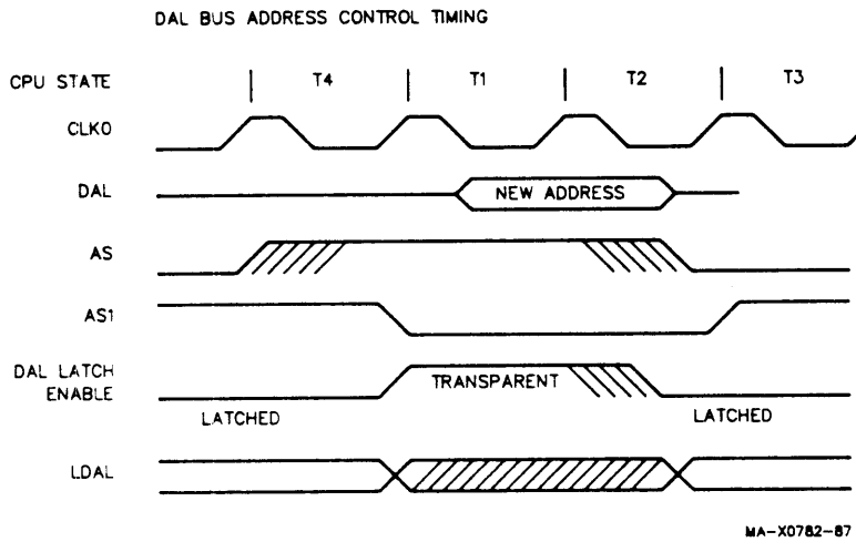
Figure A-1: DAL Bus Address Control
