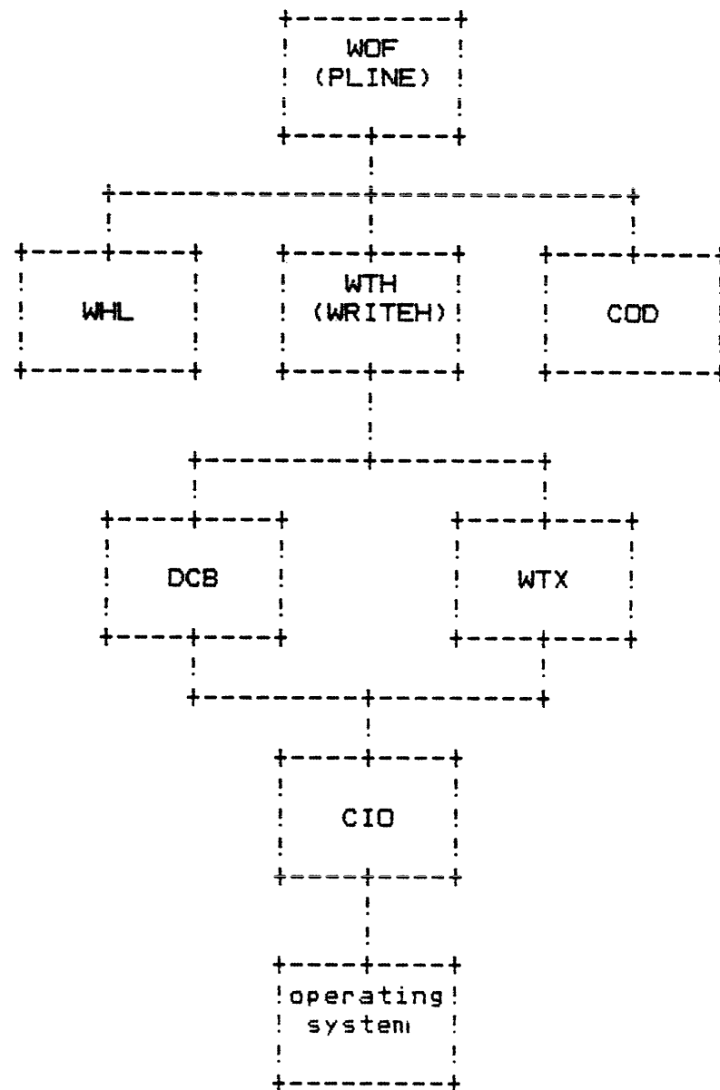
Fig. 3.11. Write routines hierarchy - (CIO)
