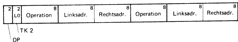
Bild 2e Befehlspar - Zweiadressenbefehle
