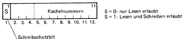
Bild 12 Viertelwort in Seiten-Kachel-Tabelle
