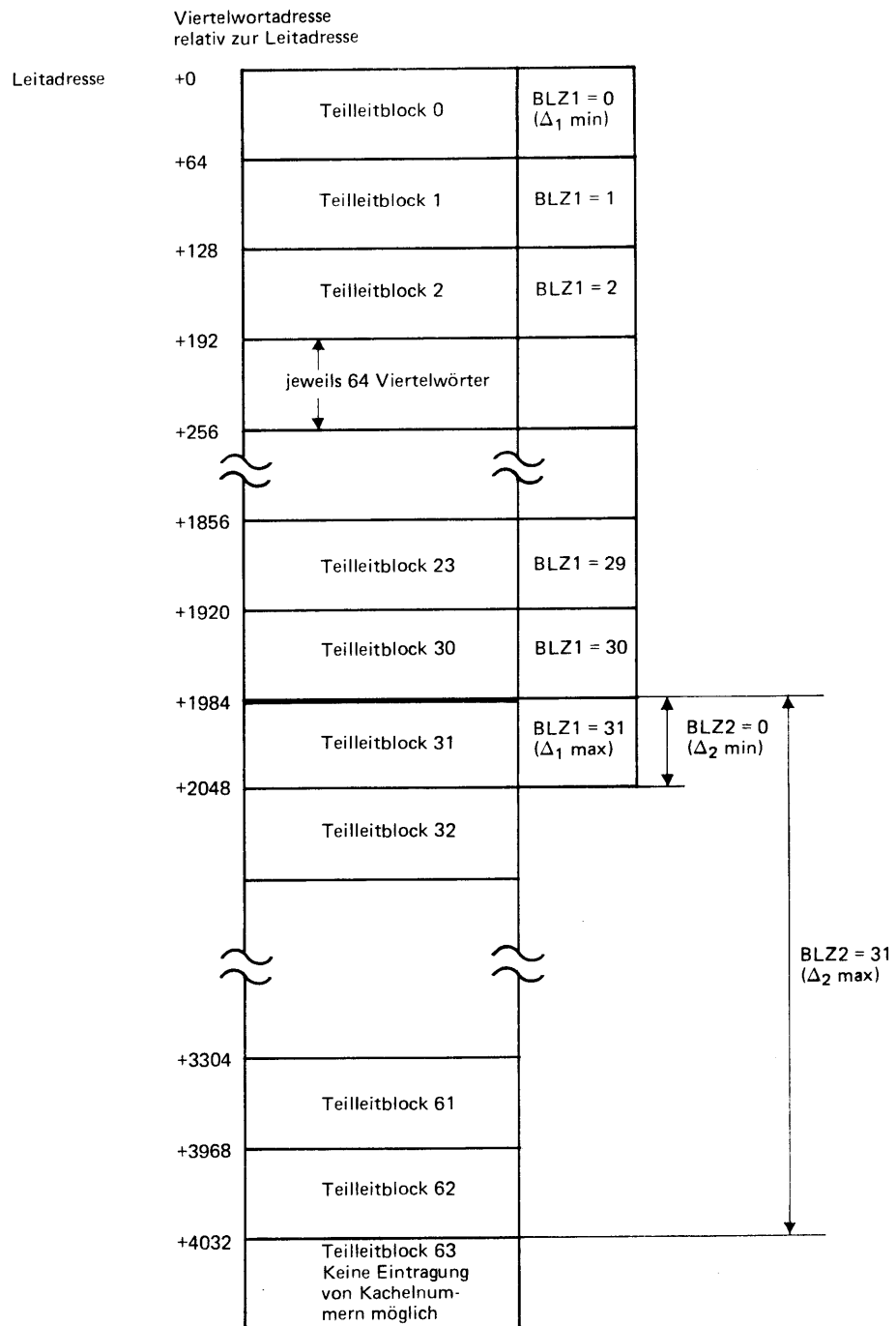
Bild 13 Aufteilung des Prozeßleitblocks in Viertelworte
