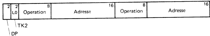
Bild 2d Befehlspar - Einadressenbefehle
