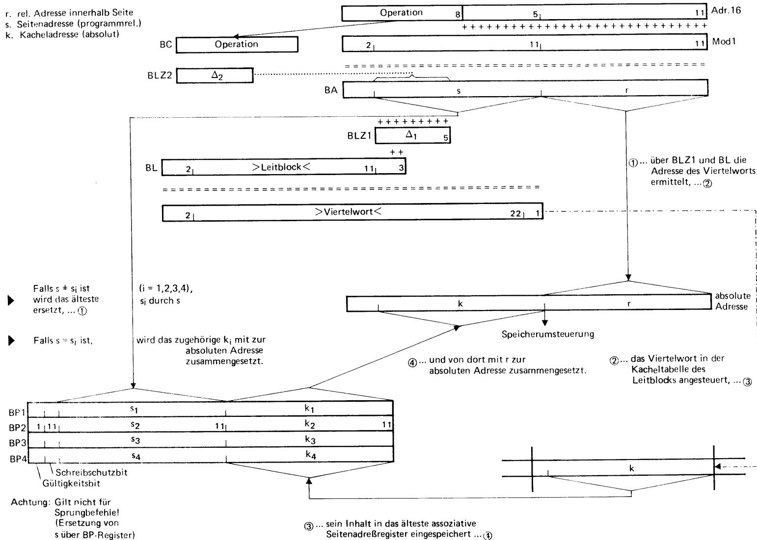
Bild 16 Ersetzung der programmrelativen 16-Bit-Adresse mit der Kacheladresse
